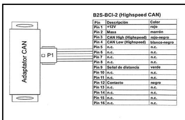
Figura 9. Especificaciones adaptador Beijer (HALE).
