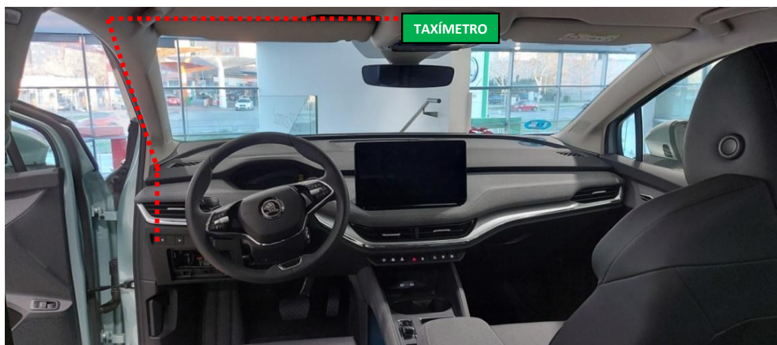
Figura 16. Recorrido de la manguera del taxímetro.
