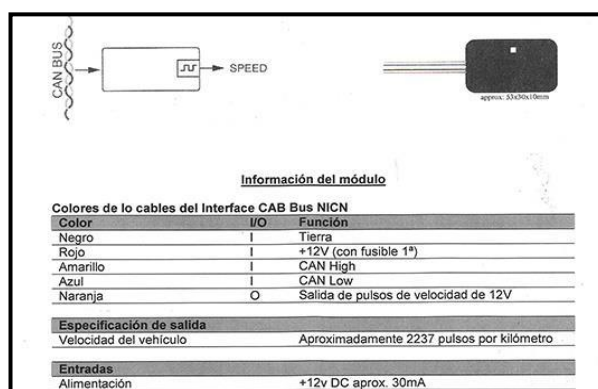
Figura 10. Especificaciones adaptador Nitax.
