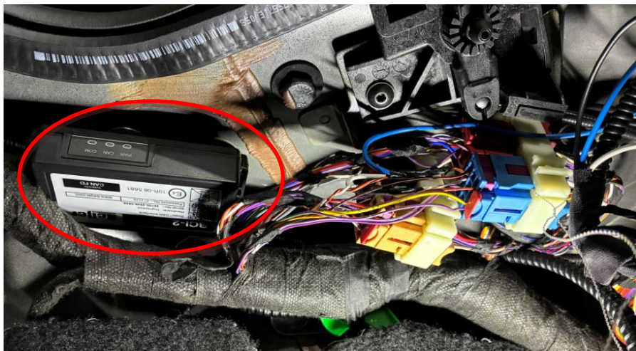
Figura 11. Ubicación del adaptador de CAN-BUS.
