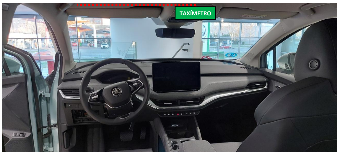
Figura 18. Trazado del cable del módulo tarifario.
