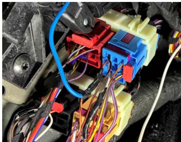
Figura 6. Conector de la unidad de control de la red de abordo (azul).
