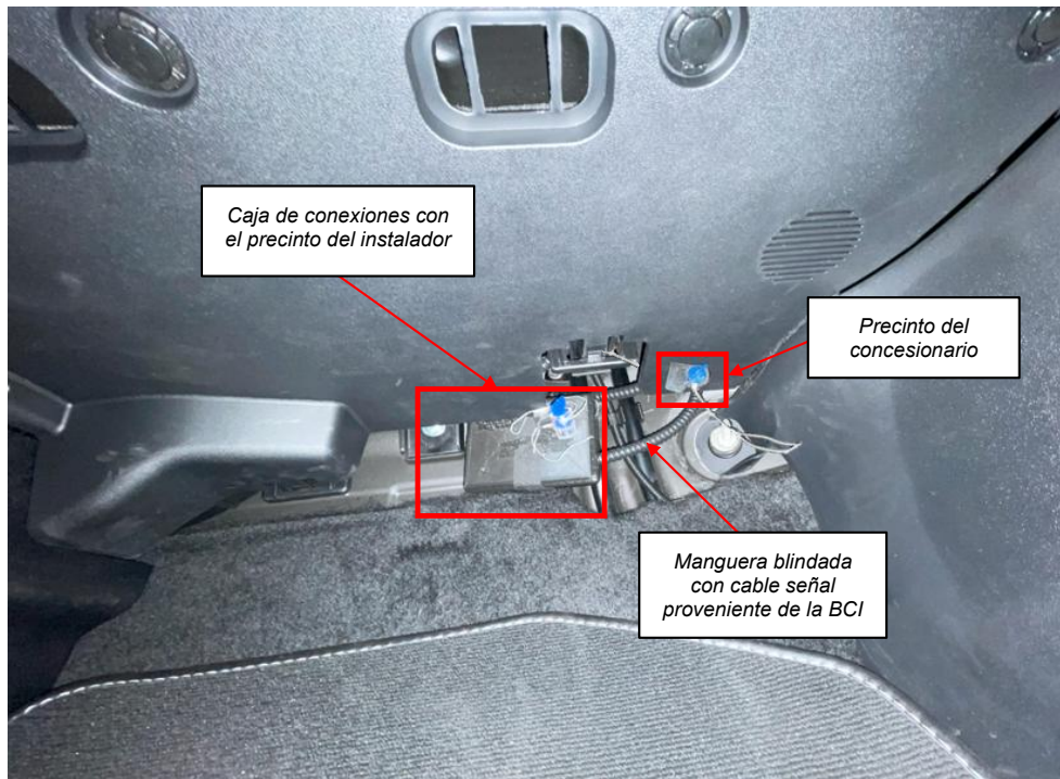
Figura 4.1.1.1: Ubicación prevista para la caja de conexiones
