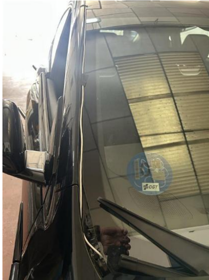
Figura 4.2.4.8. Recorrido del cable del módulo por el vierteaguas
