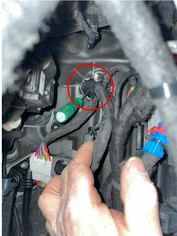
Figura 4.2.4.11. Vista del pasamuros desde el interior
