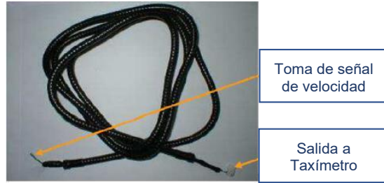
Figura 3.1.1.1: Ejemplo de manguera para señal de velocidad
