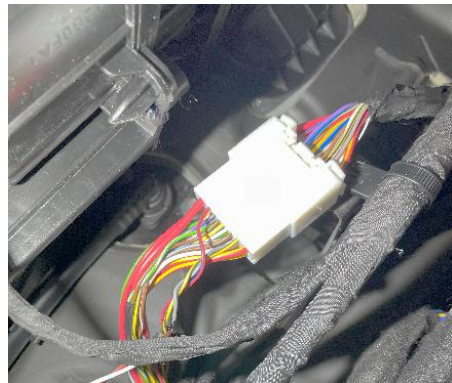
Figura 3.3.1.2. Vista del conector FBBDR
