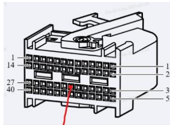
Figura 3.3.1.5. Via 33 del conector BD526
