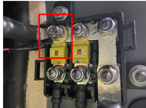
Figura 3.3.2.13. Positivo directo de batería (+30)
