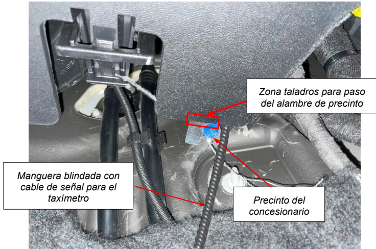
Figura 3.3.3.1: Vista del precintado efectuado por del concesionario
