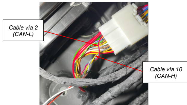
Figura 3.3.2.8. Empalmes de la señal CAN Bus
