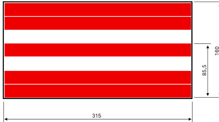
Figura 4.2.4.5. Posición y longitud de las tiras de cinta adhesiva de doble cara
