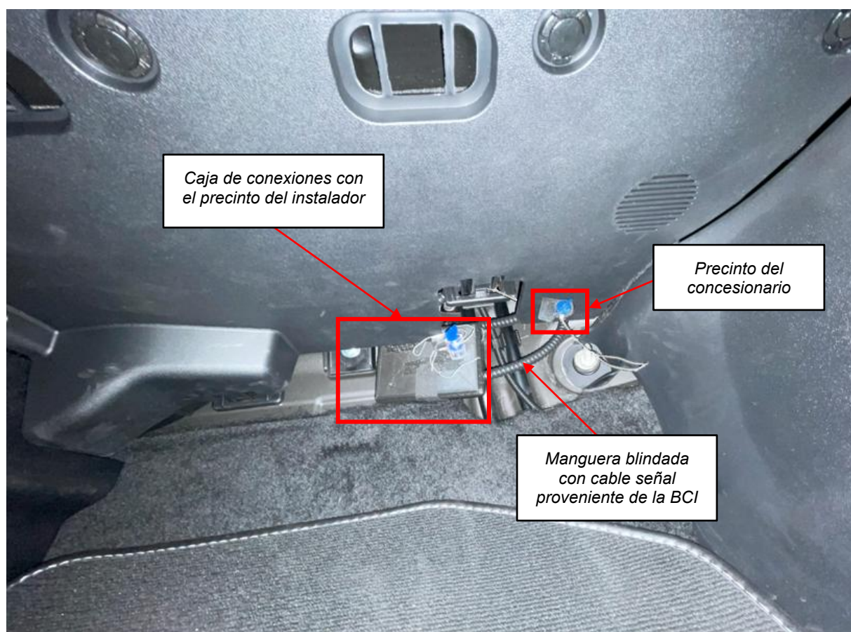
Figura 4.1.1.1: Ubicación prevista para la caja de conexiones
