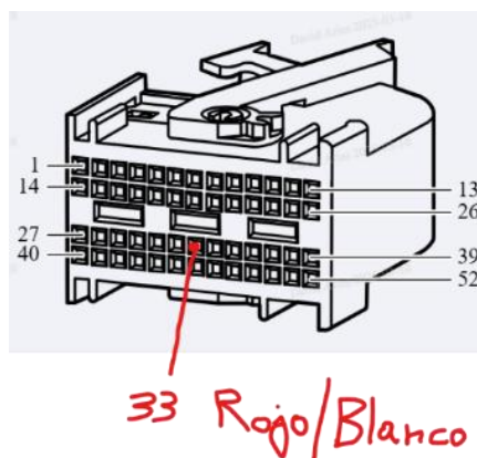
Figura 3.3.1.5. Vía 33 del conector BD526
