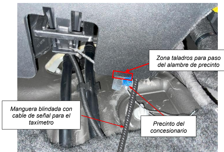
Figuras 3.3.3.1: Vista del precintado efectuado por el concesionario
