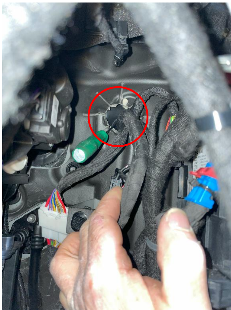
Figura 4.2.4.11. Vista del pasamuros desde el interior
