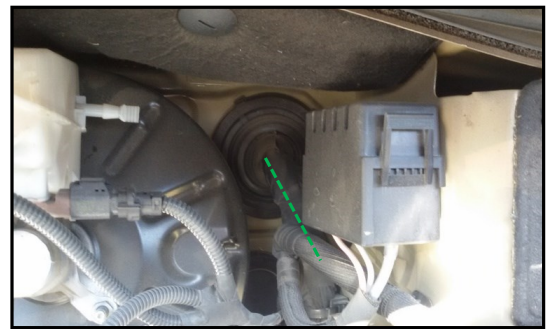
Recorrido de los cables a través del pasamuros del motor
