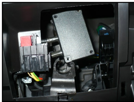
Caja de señales en la cubierta inferior bajo volante
