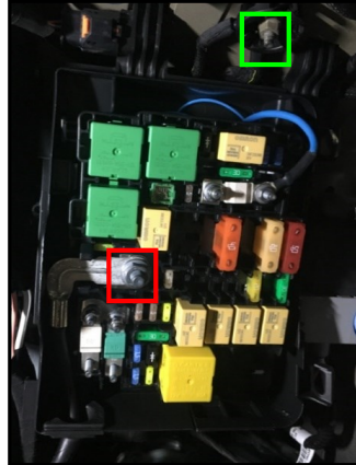
Caja fusibles tipo 2
