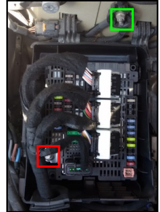
Caja fusibles tipo 3
