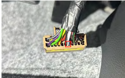
Figura 3.3.1.4: Identificación del pin 18
