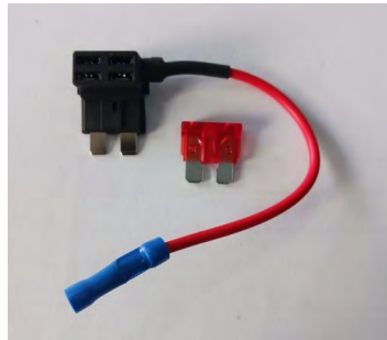
Figura 4.1.2.1: Ejemplo de roba fusibles
