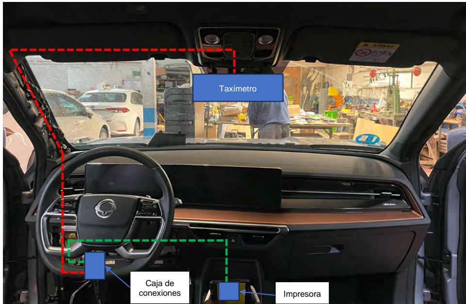
Figura 4.2.4.1: Esquema general de conexiones
