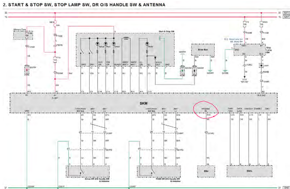
Figura 3.3.1.3: Esquema eléctrico de la SKM
