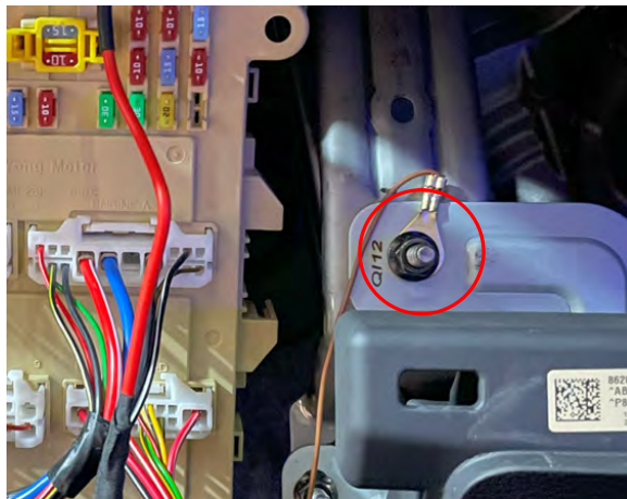
Figura 4.2.3.3: Toma de masa
