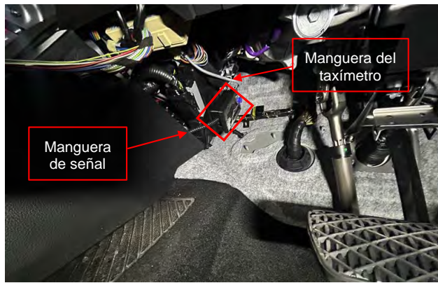
Figura 4.1.1.1: Ubicación prevista para la caja de conexiones
