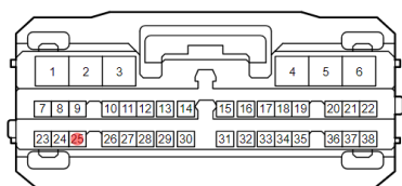
Vista frontal conector F10
