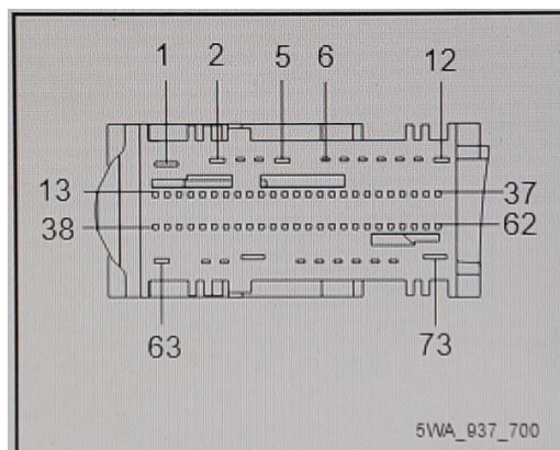
Figura 7. Esquema Clema A de 73 pines de la unidad de control de la red de abord.
