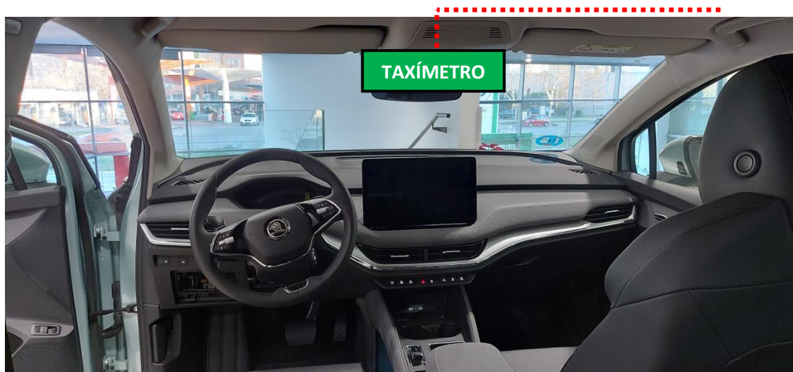
Figura 19. Trazado del cable del módulo tarifario.
