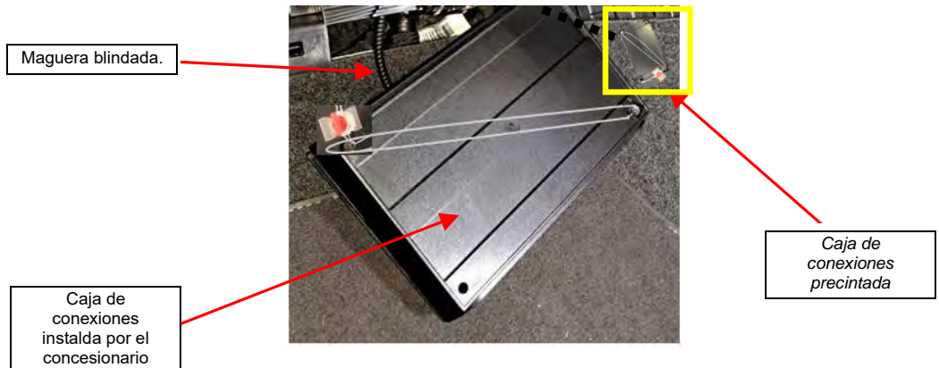
Fig. 3.1.1. Vista del de la caja de conexiones precintada e instalada con velcro.
