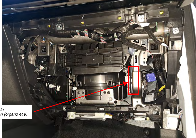
Fig. 1.10. Vista módulo guantera retirado.
