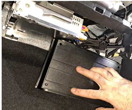
Fig.2.2.5. Detalle emplazamiento caja contenedora con manguera blindada.
