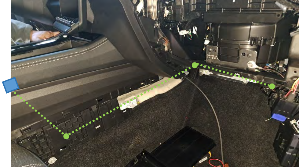
Fig. 5.1.2. Recorrido de cable de conexión impresora.
