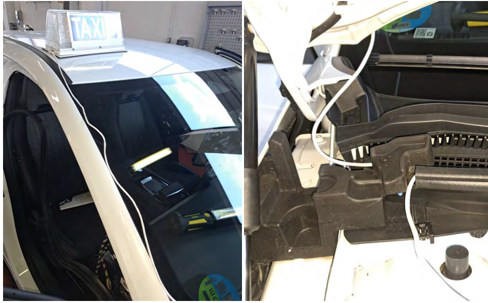
Fig. 6.2.4. Recorrido de los cables por vierteaguas del pilar A derecho.
