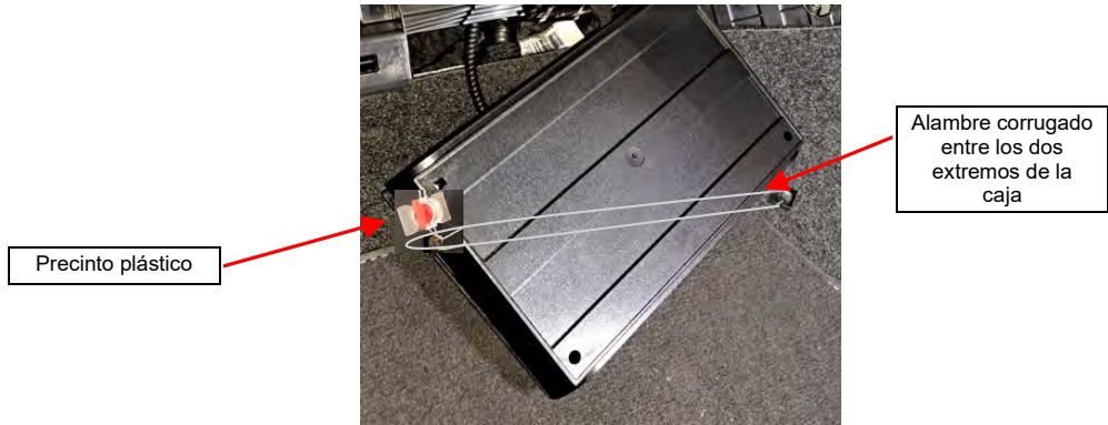
Fig.2.2.4. Detalle precintado con precinto plástico.
