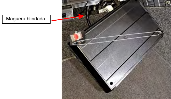
Fig.2.2.6. Detalle emplazamiento caja contenedora precintada.
