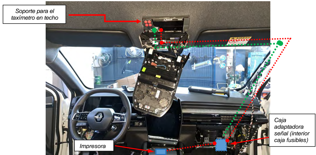
Fig. 4.2.1. Esquema orientativo de las conexiones.
