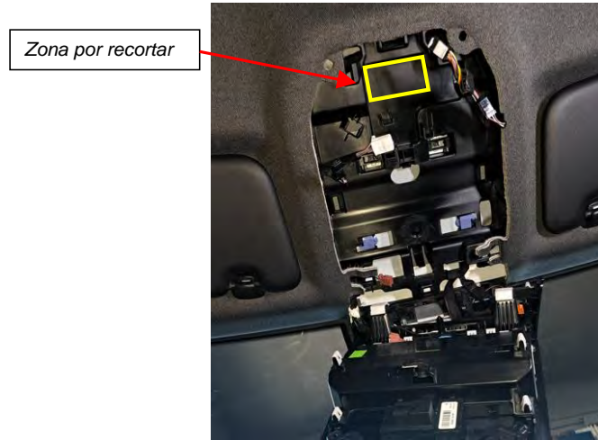
Fig. 6.1.1 Vista zona bajo plafón delantero..
