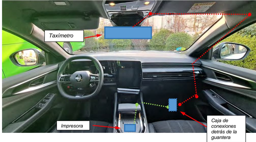
Fig. 4.1. Esquema orientativo de las conexiones.
