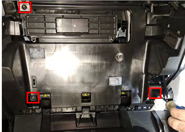
Fig. 1.7. Retirar los 3 tornillos marcados.
