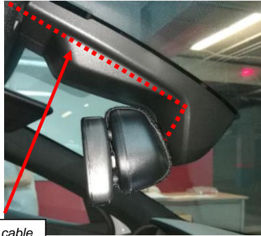
Recorrido cable Taxímetro
