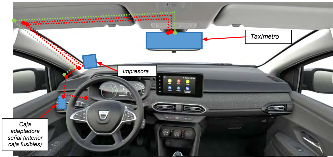
Fig. 4.4. Esquema orientativo del recorrido de las conexiones para taxímetros de espejo (SEÑAL ANALÓGICA)
