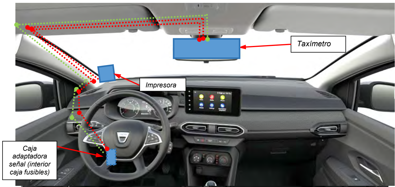
Fig. 4.5. Esquema orientativo del recorrido de las conexiones para taxímetros de espejo (SEÑAL DIGITAL)
