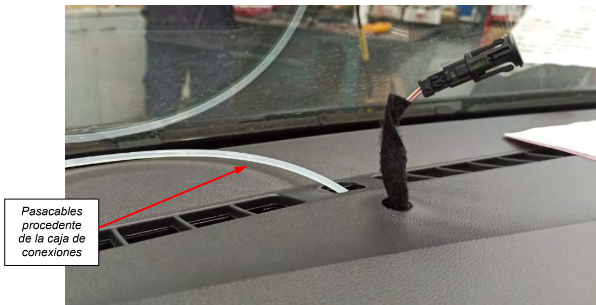
Fig. 4.3. Vista del paso de la manguera a la zona superior del salpicadero.
