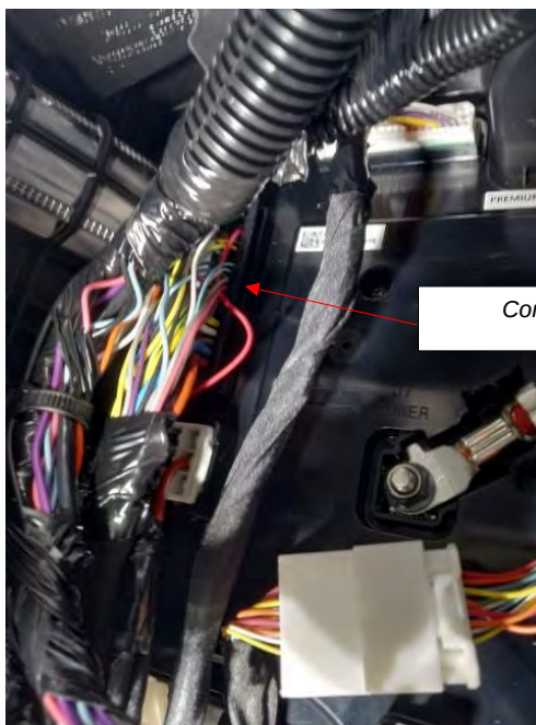
Esquema del emplazamiento del conector X030
