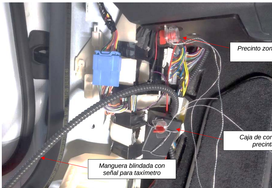
Vista genera del conjunto de conexiones
