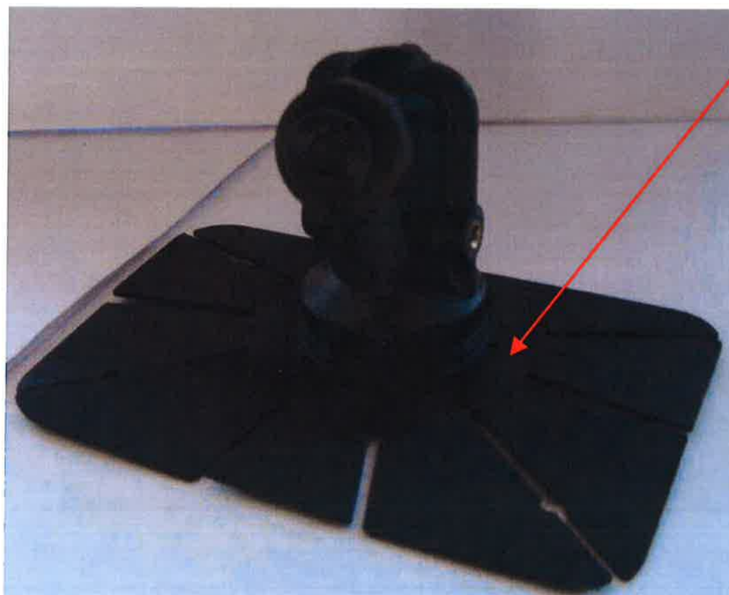
Fig. 11.2. Vista de un ejemplo de soporte de plástico para taxímetro.
