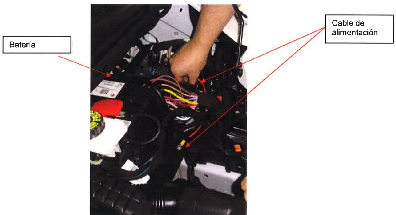
Fig. 4.2. Fotografía de los puntos para la toma de alimentación.
