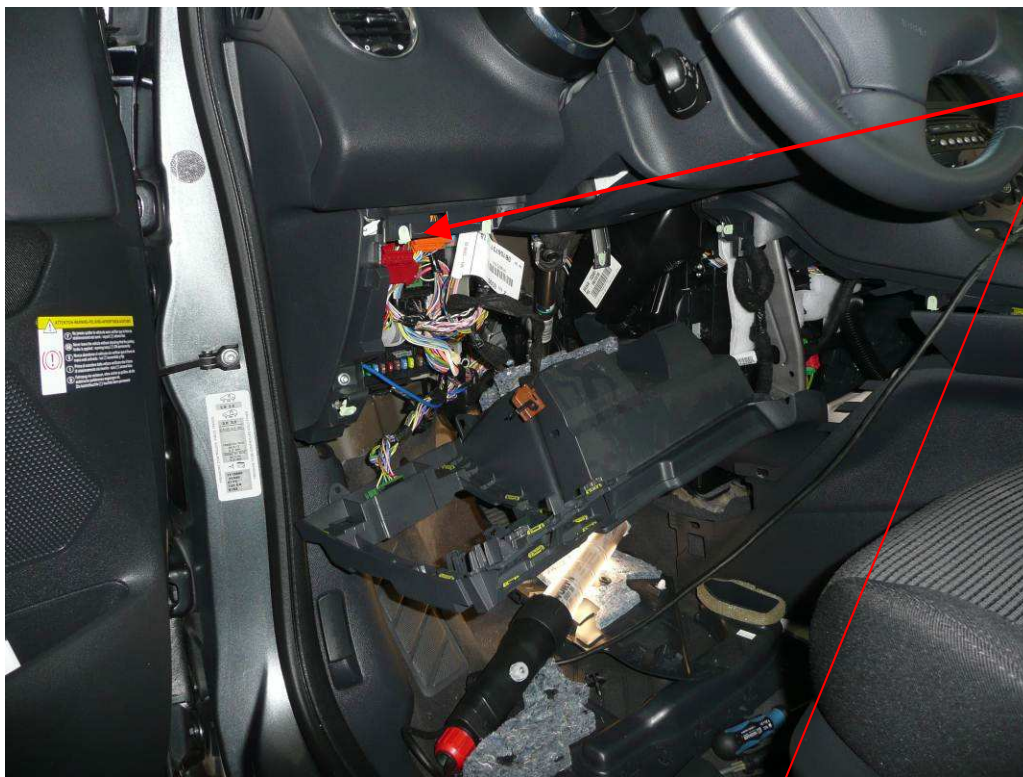
Fig. 1.3. Vista detalle de la caja de fusibles y conector IC01.
