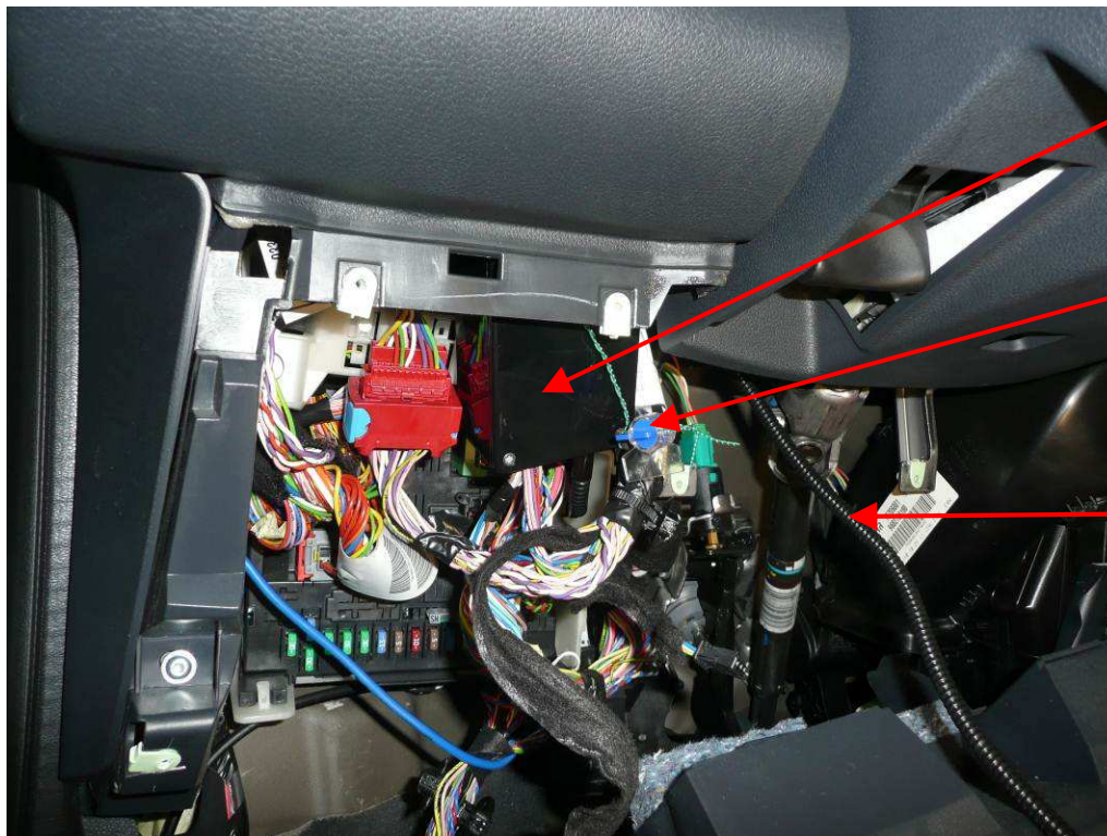
Fig. 3.4. Inserción de la caja precintada en el interior del compartimento de conexiones
