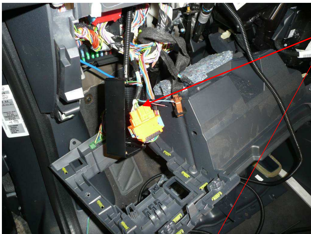
Fig. 2.1. Vista del conector IC01 extraído. La señal se obtendrá de la parte trasera.
