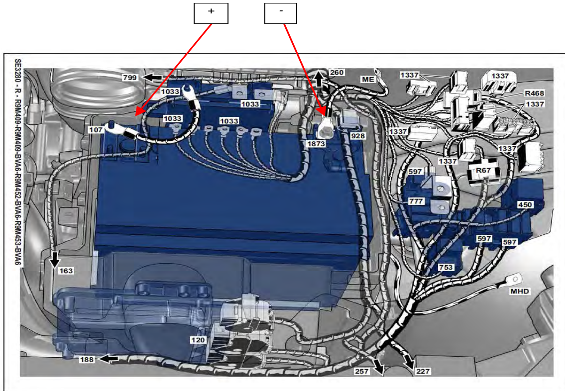
Fig. 1.9. Esquema de la batería.
