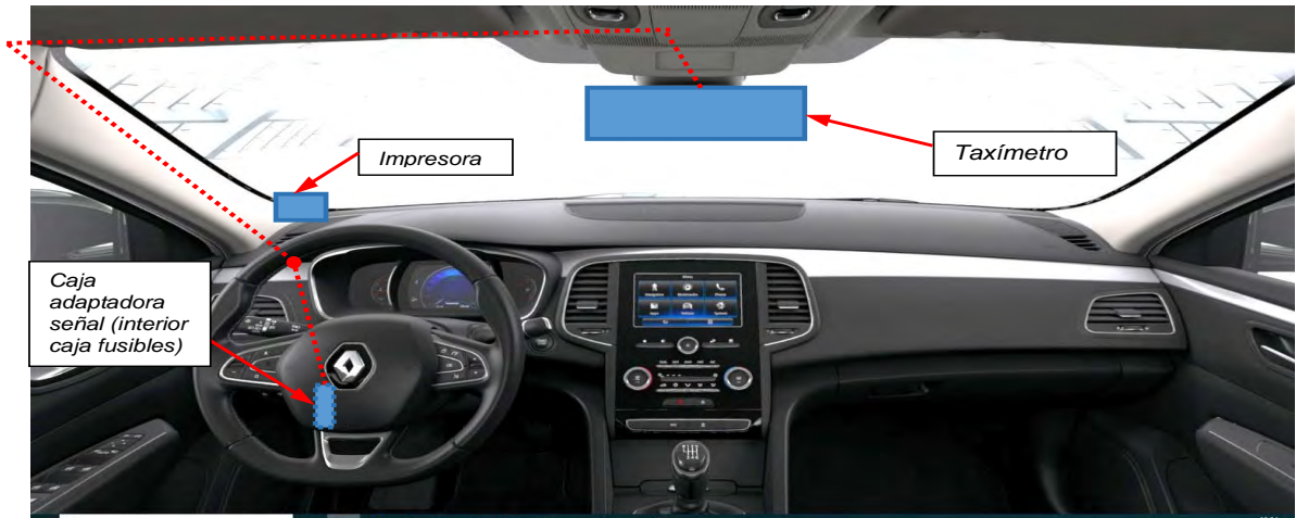
Fig. 4.4. Esquema orientativo de las conexiones.
