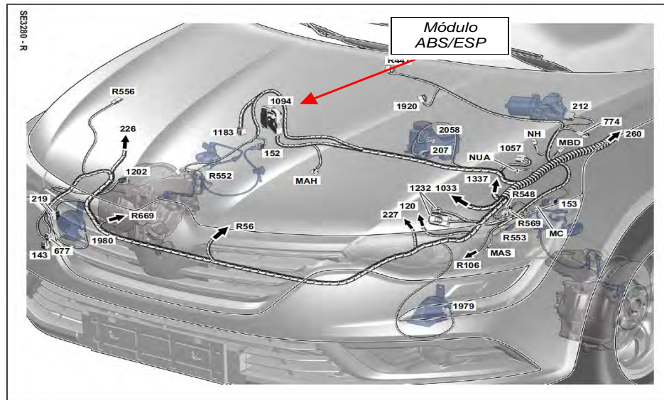
Fig. 1.2. Esquema general de conectores
