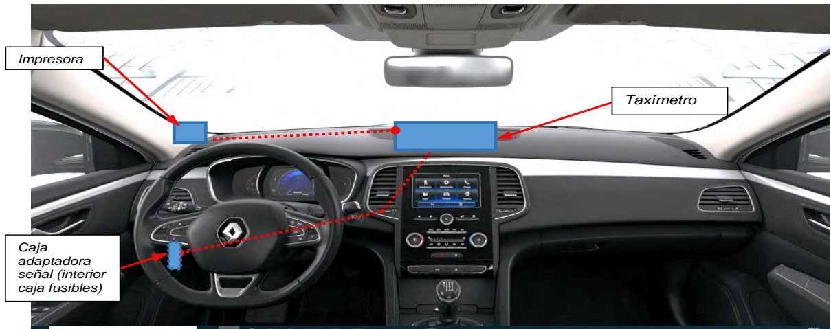
Fig. 4.1. Esquema orientativo del recorrido de las conexiones para taxímetros sobre salpicadero .
