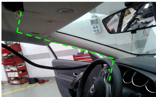
Fig. 10.1.3. Vista recorrido del cableado entre el módulo y la caja adaptadora de señal
