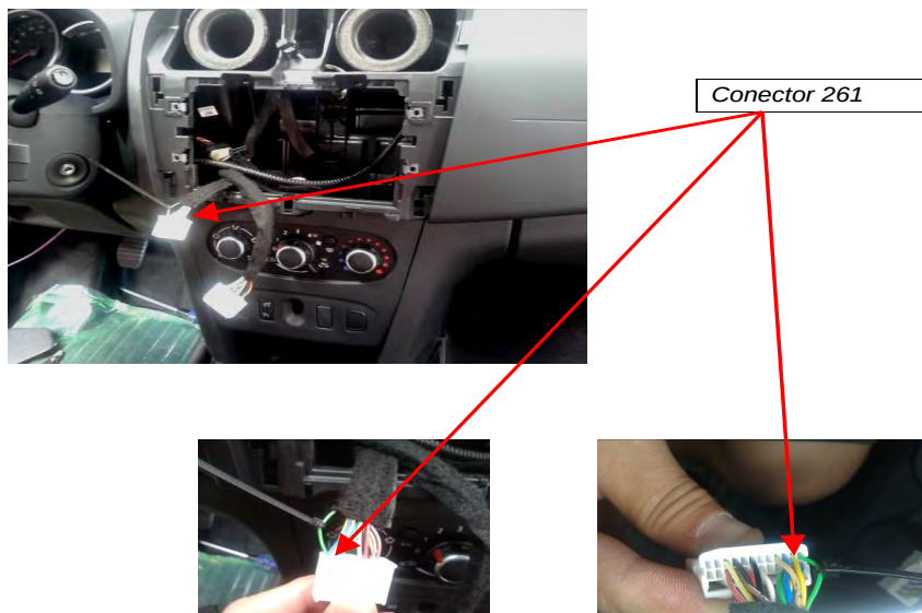
Fig. 2.1. Vista de la ubicación del conector 261.
