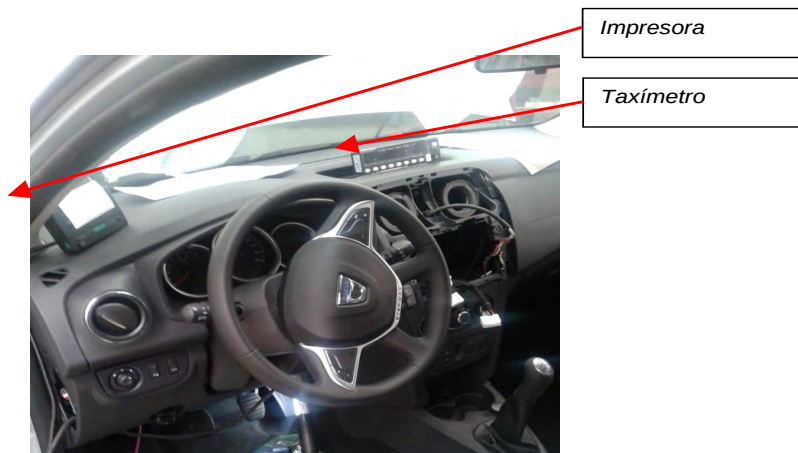
Fig. 5.2. Vistas de la disposición del taxímetro y la impresora.
