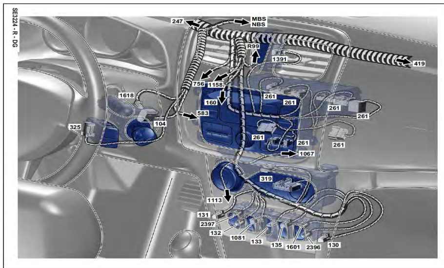
Fig. 1.2. Esquema de conectores
