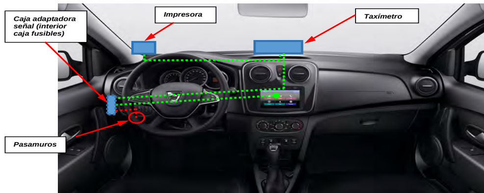
Fig. 4.1. Esquema orientativo de las conexiones.
