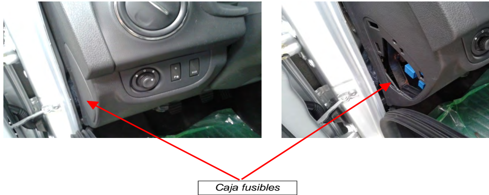
Fig. 3.1. Vista de la caja de fusibles, donde se ubicará a la caja adaptadora de conexiones.
