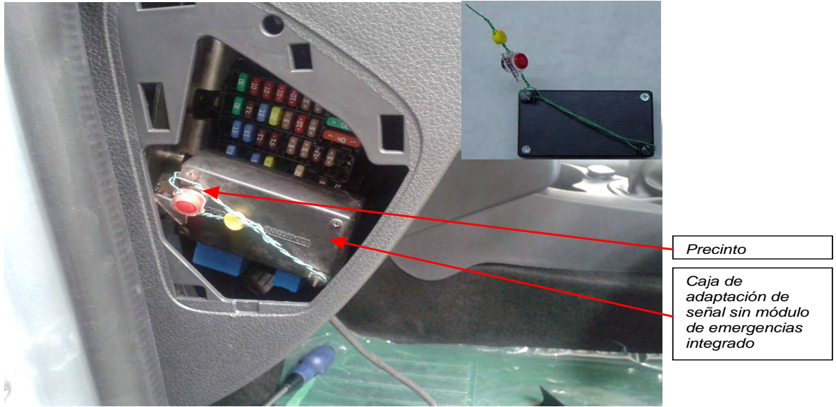
Fig. 3.2. Vistas de la caja adaptadora de señal y detalle del precinto.
