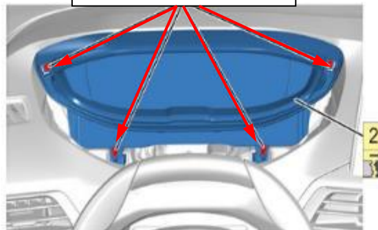
Tornillos para extracción de cuadro de instrumentos
