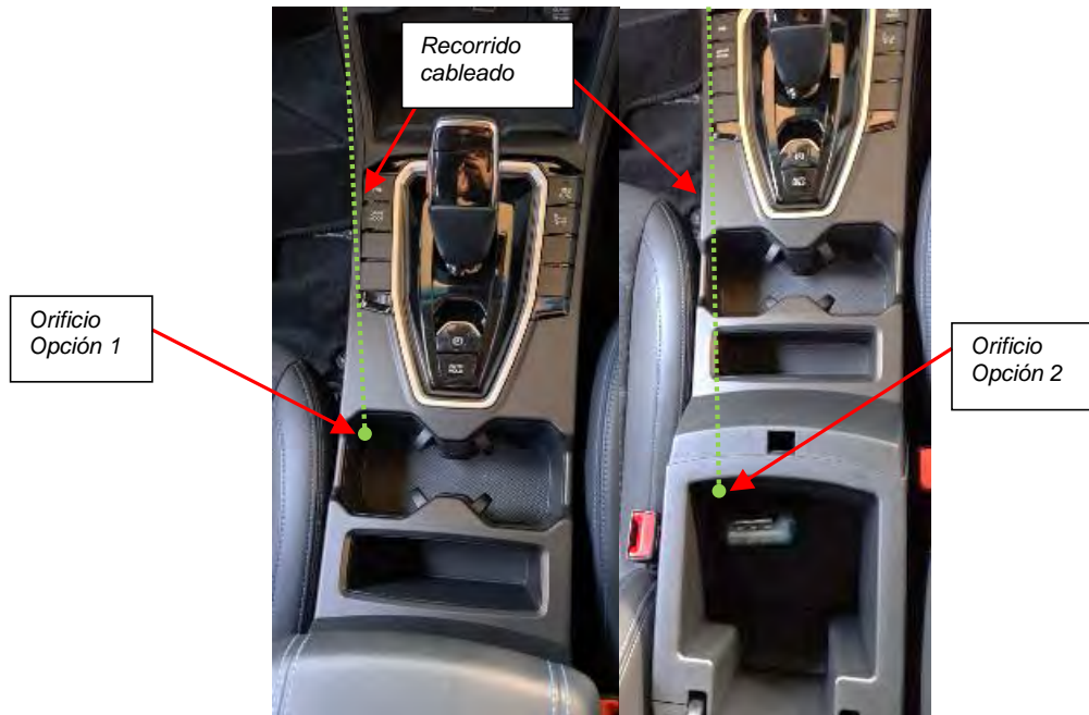
Fig. 5.3.3. Recorrido de cable Opción 1 y 2.
