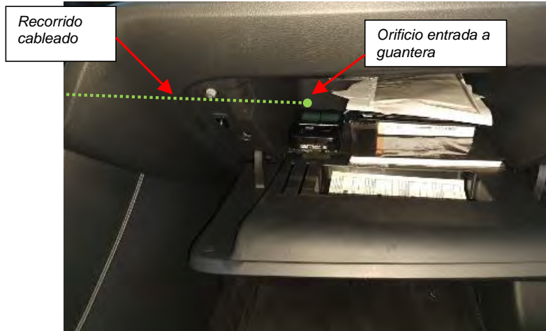
Fig. 5.3.4. Orificio para cable Opción 3.
