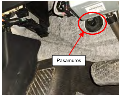
Fig. 2.1. Detalle pasamuros desde el habitáculo interior.
