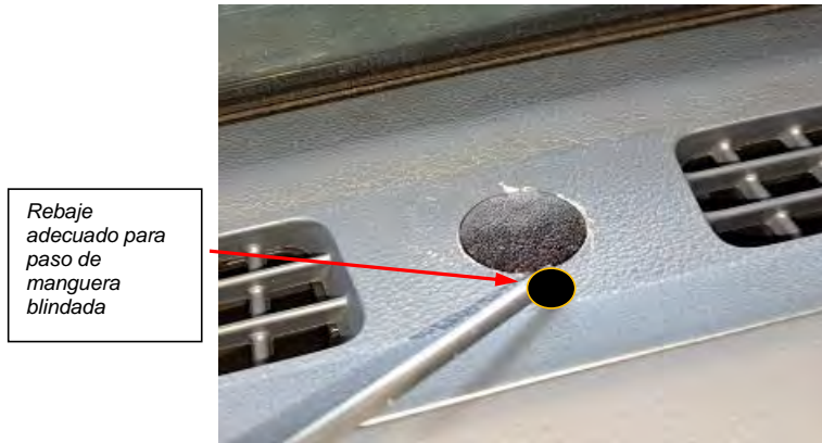
Fig. 4.1.4. Rebaje para paso de manguera blindada.
