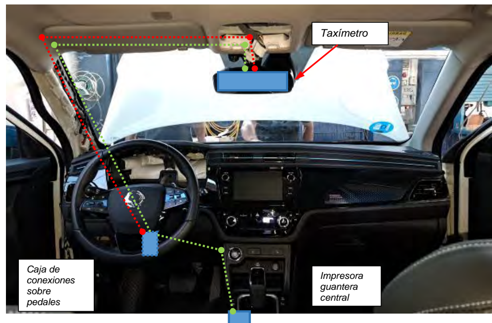
Fig. 4.2.1. Esquema orientativo de las conexiones.
