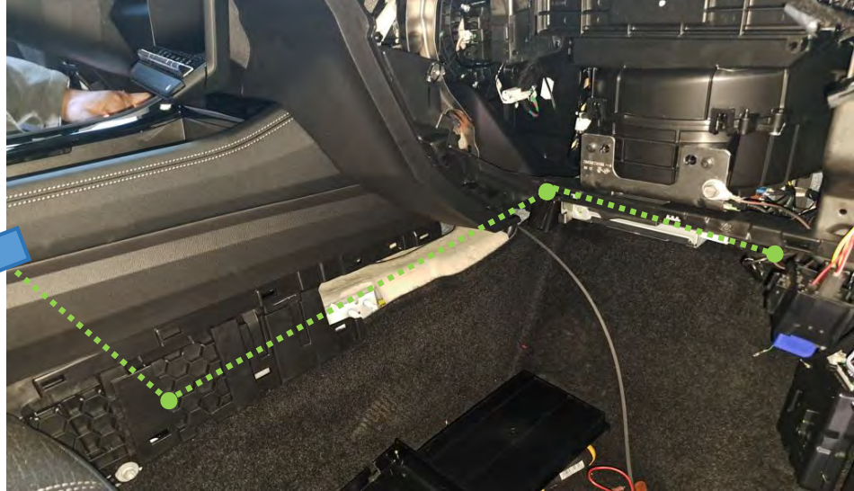
Fig. 5.1.2. Recorrido de cable de conexión impresora.
