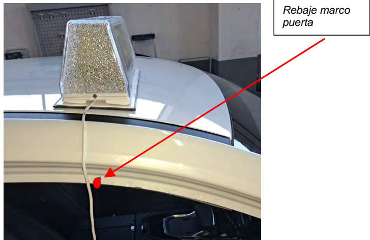
Fig. 6.2.2. Vista del módulo sobre soporte imantado
