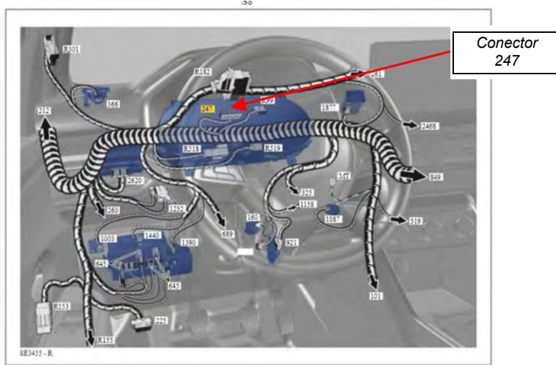
Fig. 1.1. Esquema general de conectores, zona del conductor.
