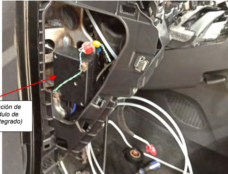
Fig. 3.3. Vista del compartimento lateral con la caja adaptadora de señal y detalle de precintos.
