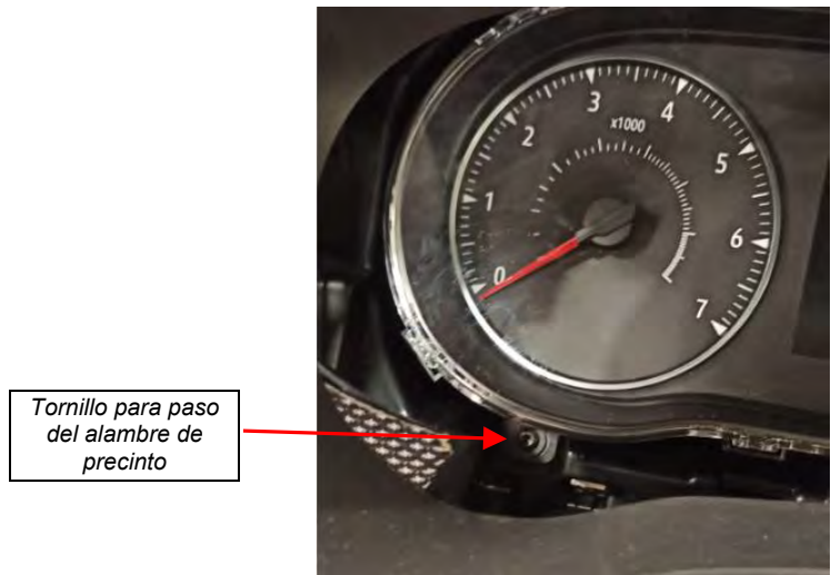
Fig. 2.4. Identificación del punto de amarre del alambre del precinto.
