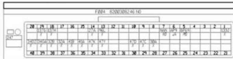
Fig. 1.3. Vista del conector 247 del cuadro de instrumentos
