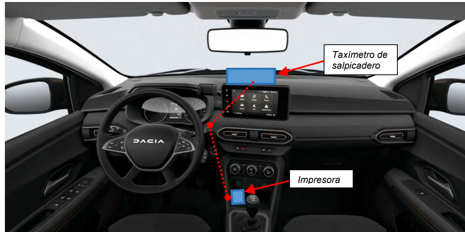
5.2.1. Recorrido cable de taxímetro de salpicadero.
