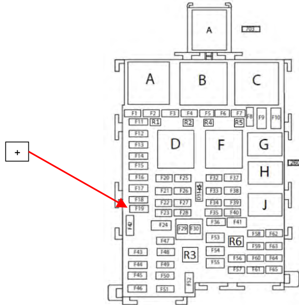
Fig. 2.4. Esquema de la Caja de Fusibles, indicando N° 23.
