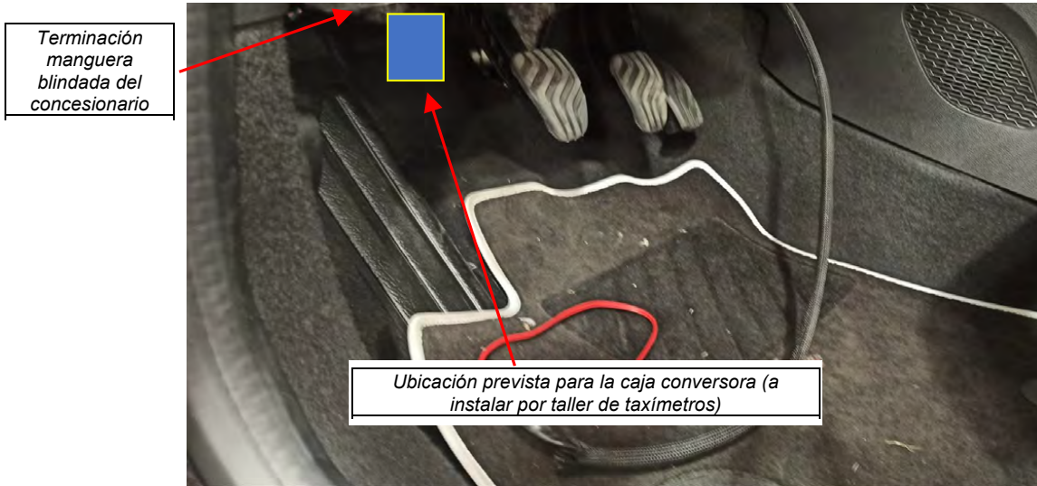
Fig. 2.2.4. Detalle ubicación de caja convertora de señal.
