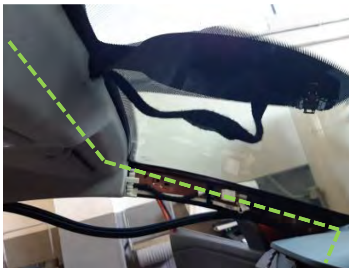
Fig. 4.2.6. Recorrido de los cables por el interior del guarnecido del marco del parabrisas.
