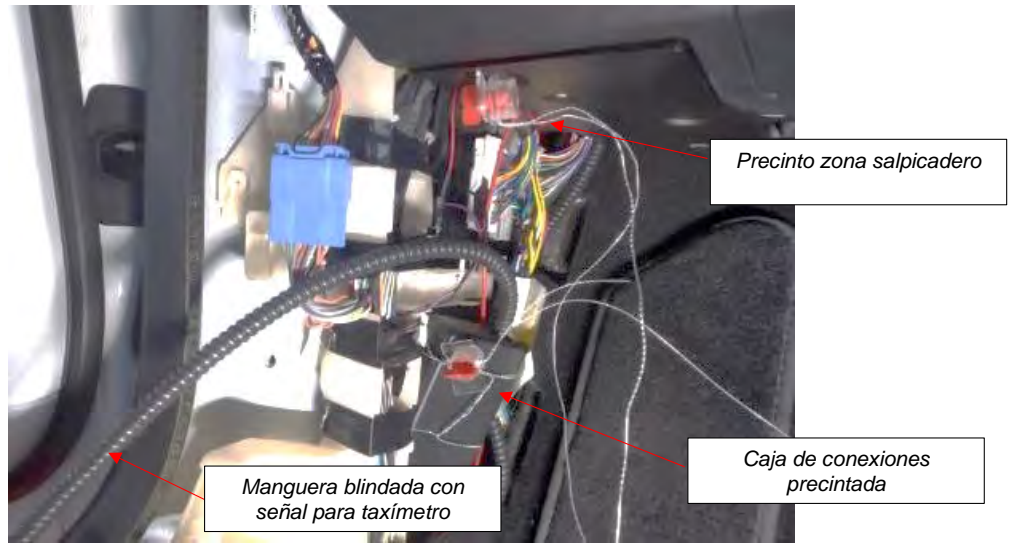
Vista general del conjunto de conexiones
