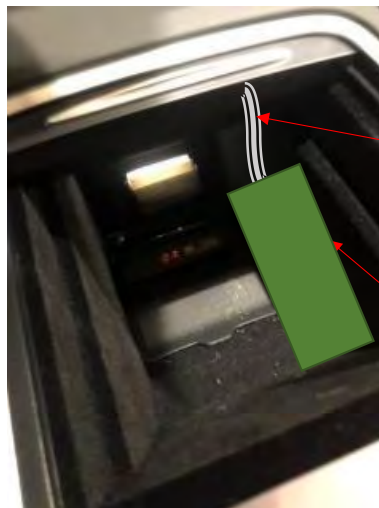
Recorrido de la manguera del cable del módulo de emergencias
