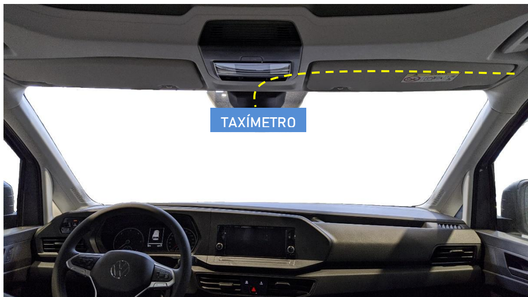
Figura 30. Trazado del cable del módulo tarifario
