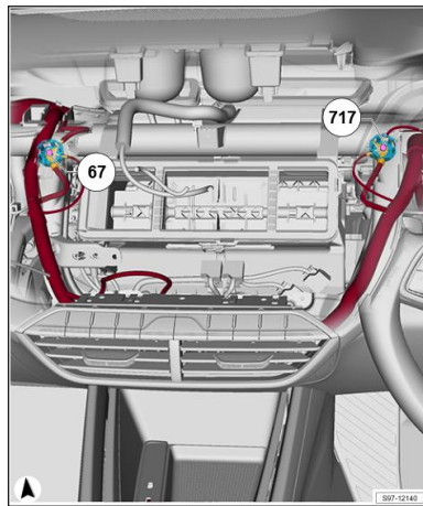
Figura 3. Punto de masa 67.
