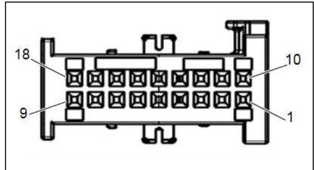
Figura 8. Detalle conexiones.
