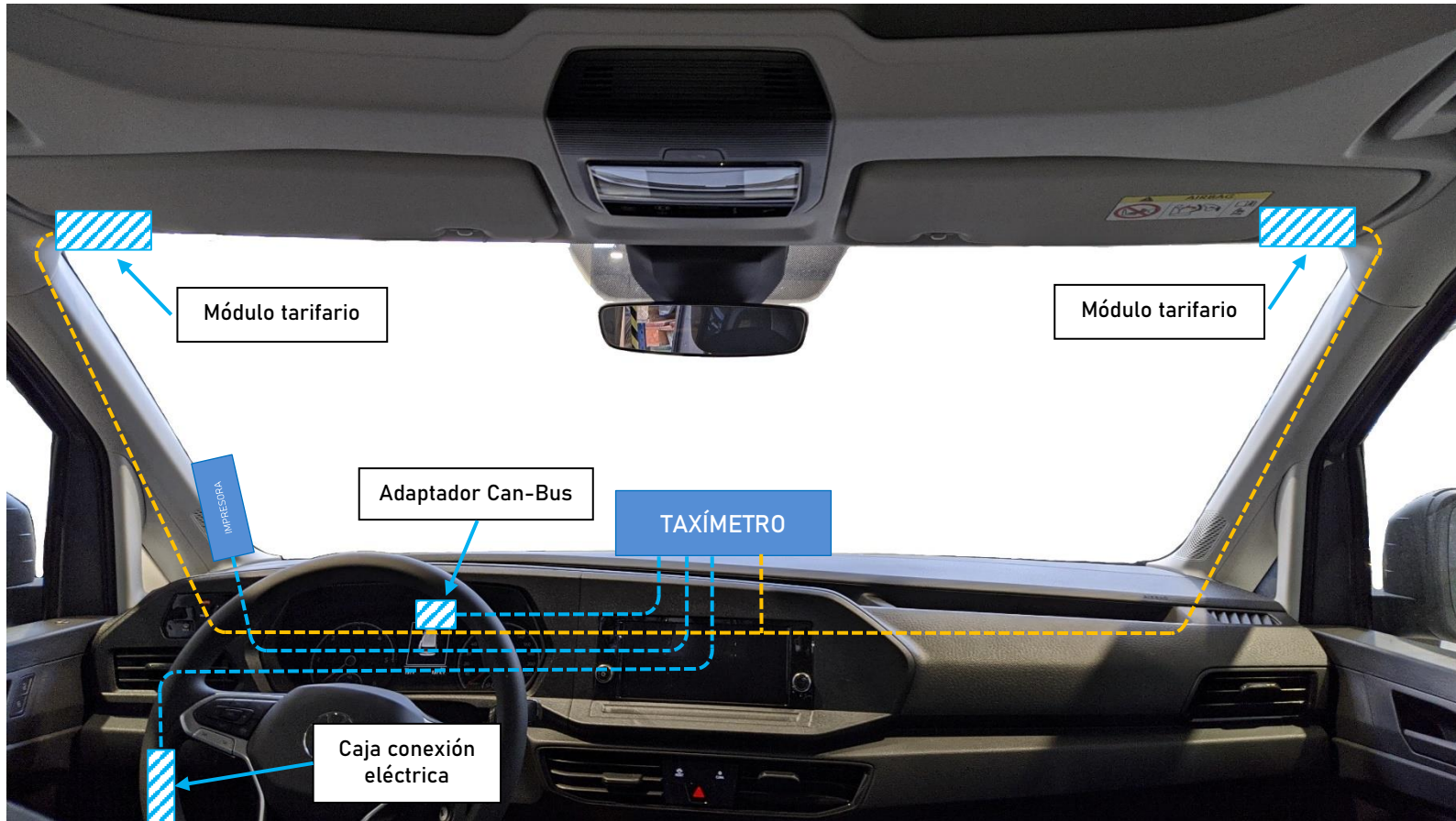
6.2. ESQUEMA DE INSTALACIÓN TAXÍMETRO CONVENCIONAL SIN CONVERTOR-ADAPTADOR DE SEÑAL (MÓDULO TARIFARIO DERECHA O IZQUIERDA)
