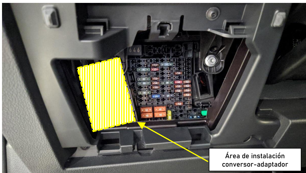
Figura 24. Área de instalación del conversor-adaptador.
