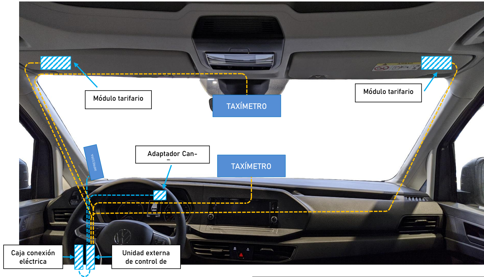
6.4. ESQUEMA DE INSTALACIÓN TAXÍMETRO CON UNIDAD EXTERNA DE CONTROL DE DATOS (TABLERO/ESPEJO) (MÓDULO TARIFARIO DERECHA O IZQUIERDA)
