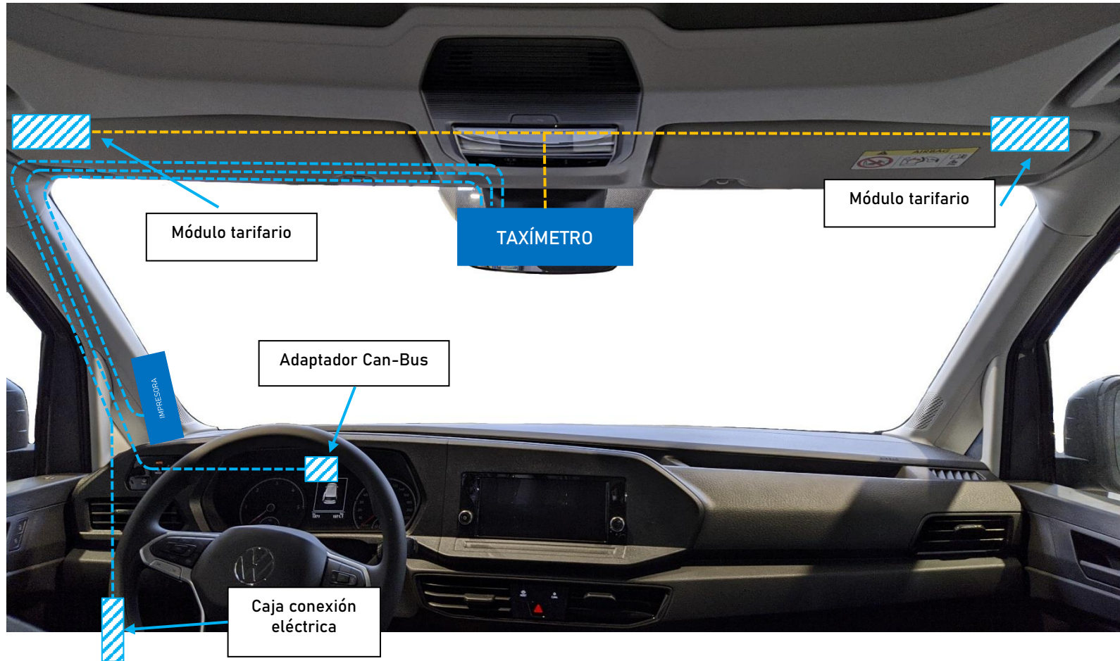
6.3. ESQUEMA DE INSTALACIÓN TAXÍMETRO EN ESPEJO INTERIOR (MÓDULO TARIFARIO DERECHA O IZQUIERDA)
