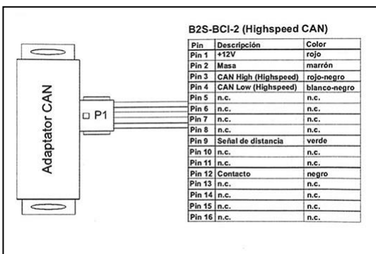
Figura 11. Especificaciones adaptador HALE.
