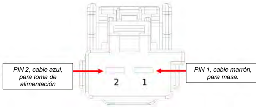
Detalle PIN del conector LV
