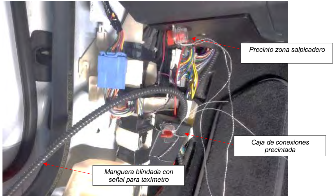
Vista genera del conjunto de conexiones
