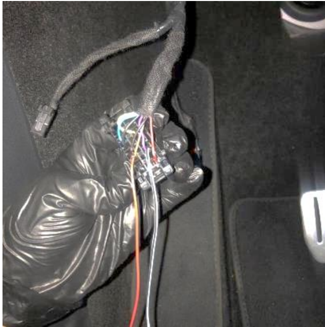
Vista de las conexiones de cables de señal sobre el conector X181
