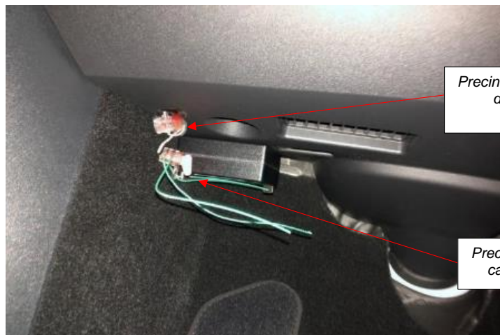
Vista final del conjunto montado y precintado TESLA, caja de conexiones superpuesta.
