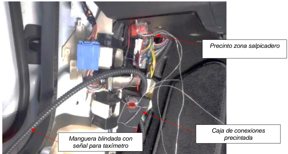
Vista general del conjunto de conexiones
