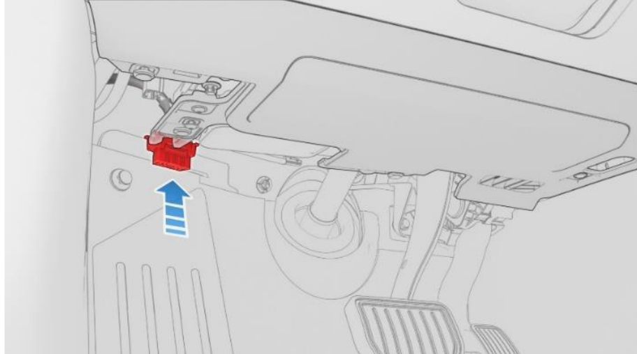
Fig. 5. Localización del conector X181
