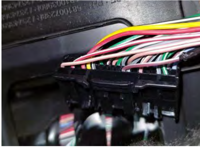
Fig. 1.3. Vista del conector 247 del cuadro de instrumentos
