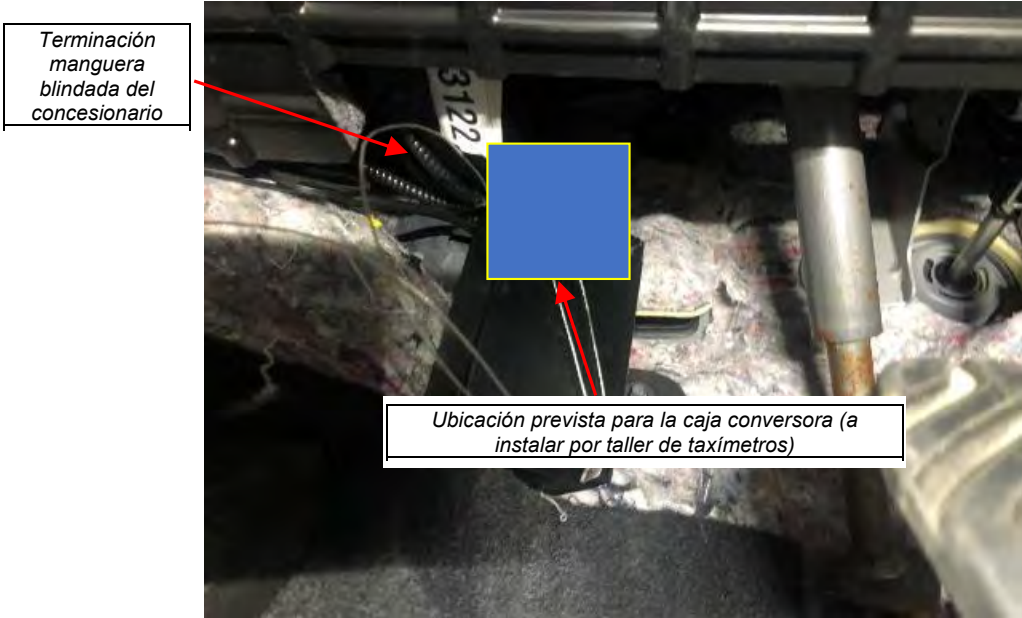
Fig. 2.2.4. Detalle ubicación de caja conversora de señal.
