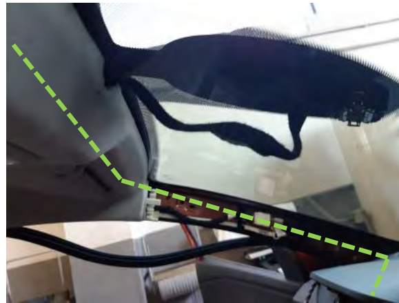
Fig. 4.2.6. Recorrido de los cables por el interior del guarnecido del marco del parabrisas.
