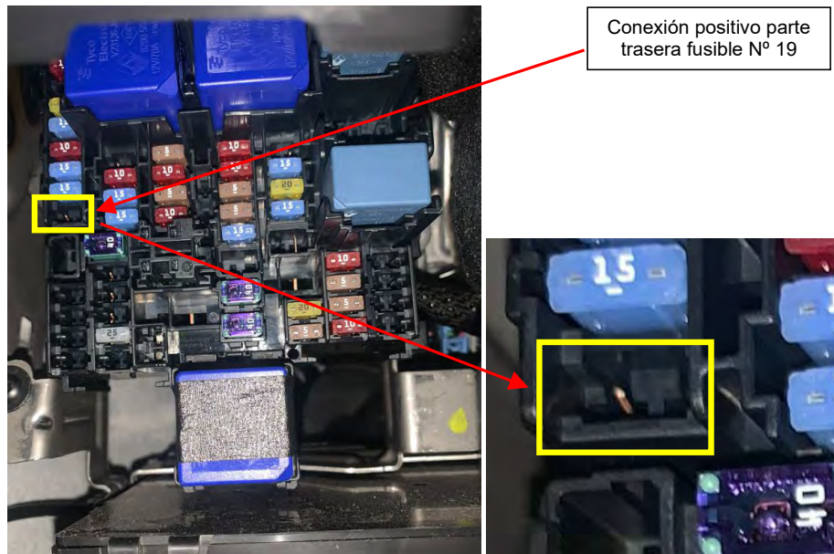
Fig. 2.5. Detalle de la Caja de Fusibles desmontada y acceso a conexión a fusible Nº 19
