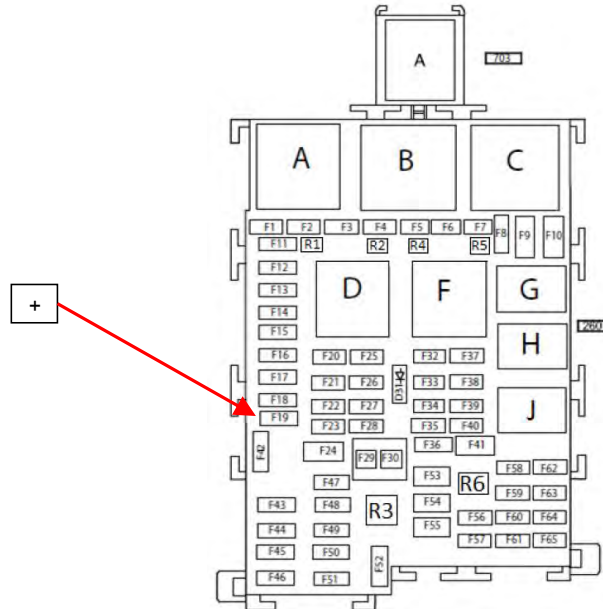
Fig. 2.4. Esquema de la Caja de Fusibles, indicando Nº 23.
