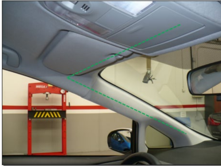
Recorrido de los cables del taxímetro de espejo
