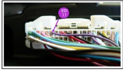
Zoom de localización del PIN 15
