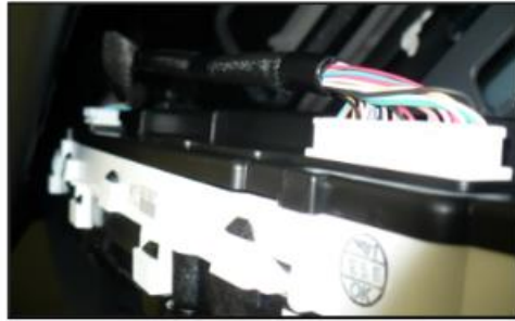
Localización del conector L27 en el cuadro
