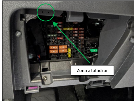
Figura 5. Zona a taladrar en el área de la caja de fusibles.
