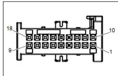
Figura 9. Detalle conexiones.
