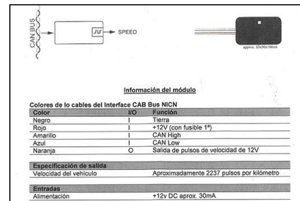
Figura 13. Especificaciones adaptador NITAX.
