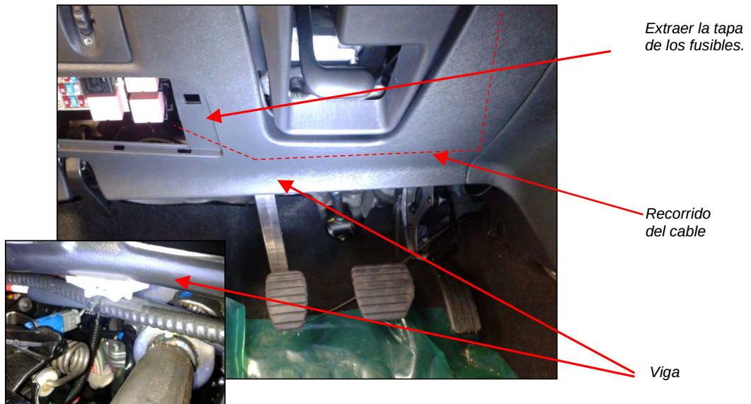
Fig. 2.2. Vista de la ubicación de la viga.
