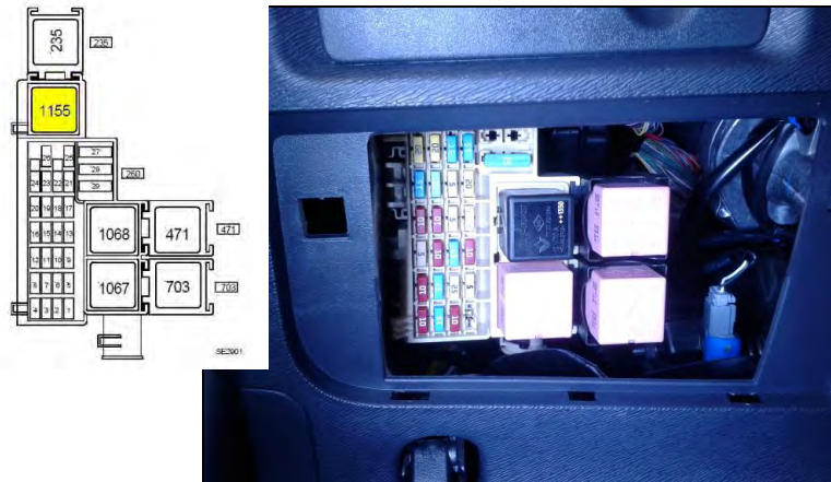
Fig. 2.1. Vista de la caja de fusibles
