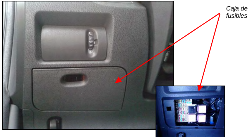
Fig. 2.1. Vista ubicación de la caja de fusibles.
