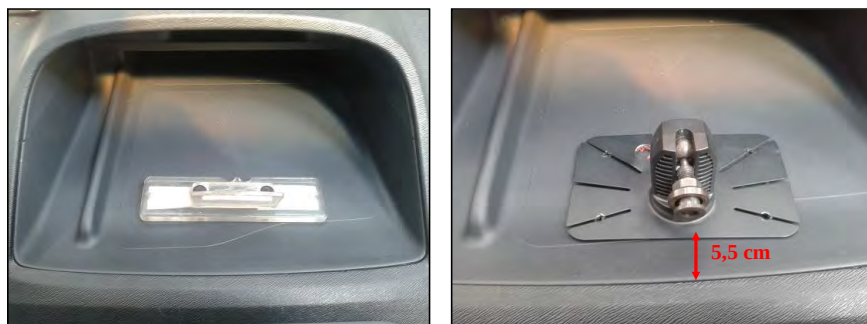
Fig. 5.2. Vistas ejemplo de soportes con cota referenciada al borde delantero del alojamiento central.
