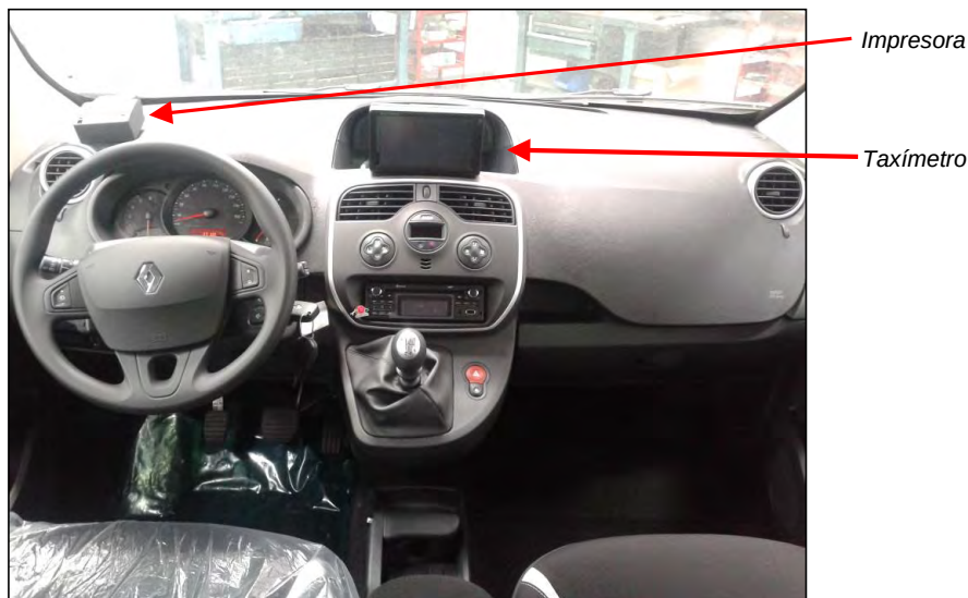
Fig. 5.3. Vistas de la disposición del taxímetro y la impresora.
