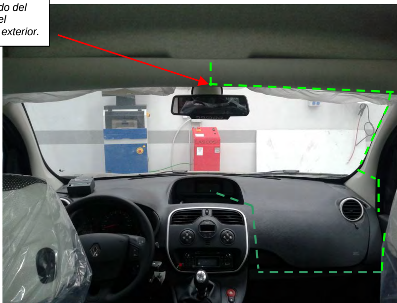
Fig. 9.2. Recorrido del cable del módulo sobre techo.
