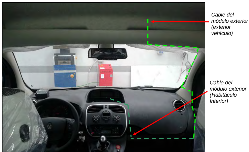
Fig. 9.6. Esquema interior cableado módulo tarifario
