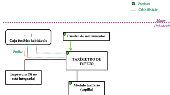
Opción 1: Sin caja de conexiones / impulsos
