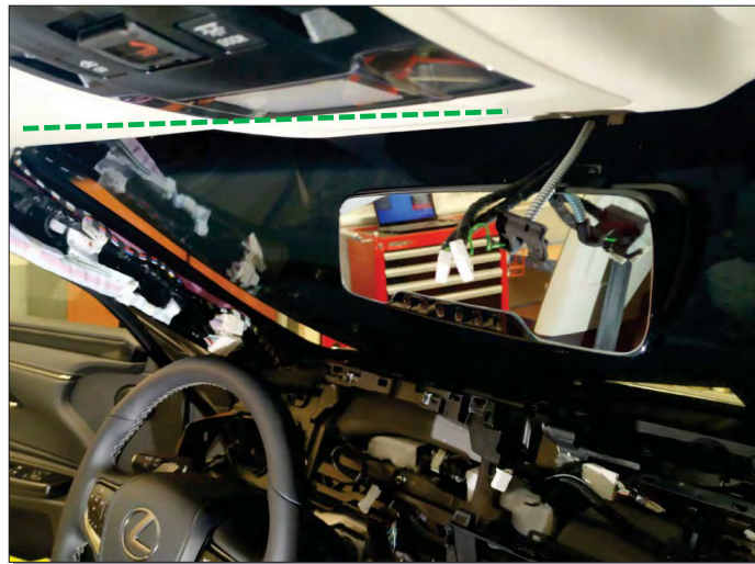
Recorrido del cable del módulo tarifario
