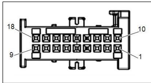
Figura 9. Detalle conexiones.
