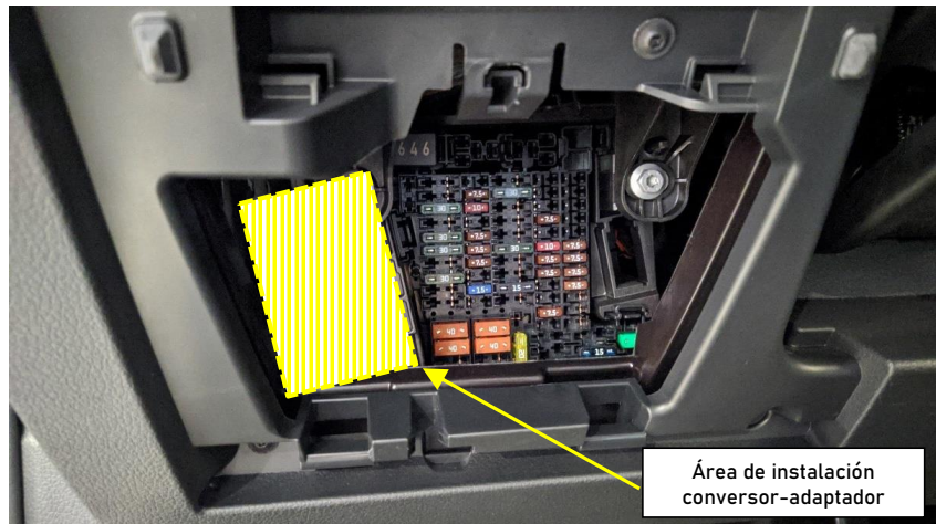
Figura 25. Área de instalación del conversor-adaptador.
