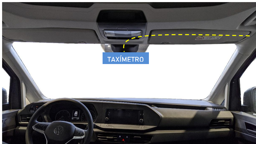
Figura 31. Trazado del cable del módulo tarifario
