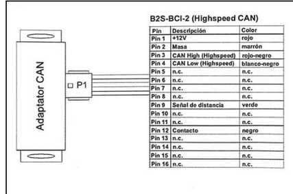
Figura 12. Especificaciones adaptador HALE.
