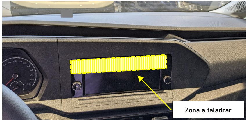
Figura 22. Zona a taladrar para el paso de mangueras.
