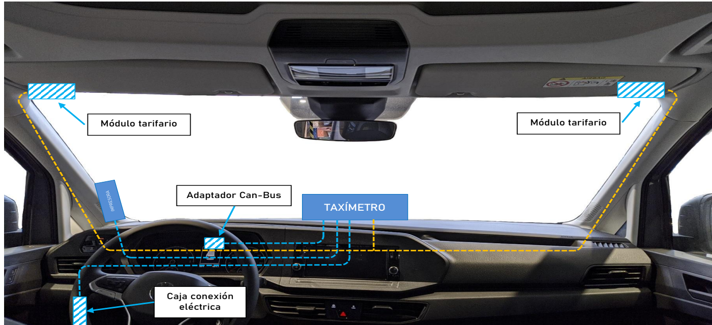
6.2. ESQUEMA DE INSTALACIÓN TAXÍMETRO CONVENCIONAL SIN CONVERTOR-ADAPTADOR DE SEÑAL (MÓDULO TARIFARIO DERECHA O IZQUIERDA)
