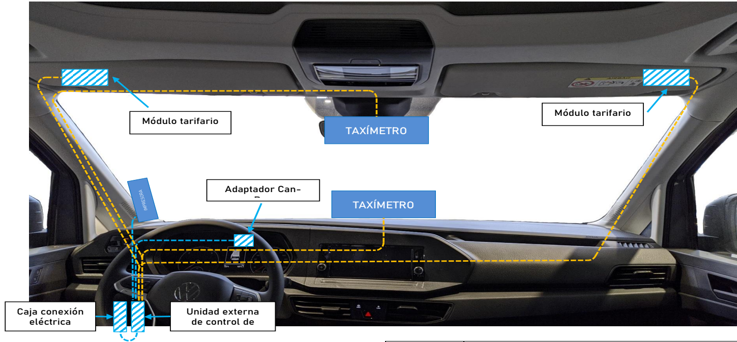
6.4. ESQUEMA DE INSTALACIÓN TAXÍMETRO CON UNIDAD EXTERNA DE CONTROL DE DATOS (TABLERO/ESPEJO) (MÓDULO TARIFARIO DERECHA O IZQUIERDA)
