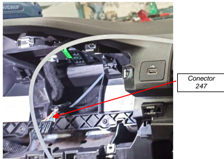
Fig. 1.2. Vista del conector 247 con el cuadro de instrumentos desmontado
