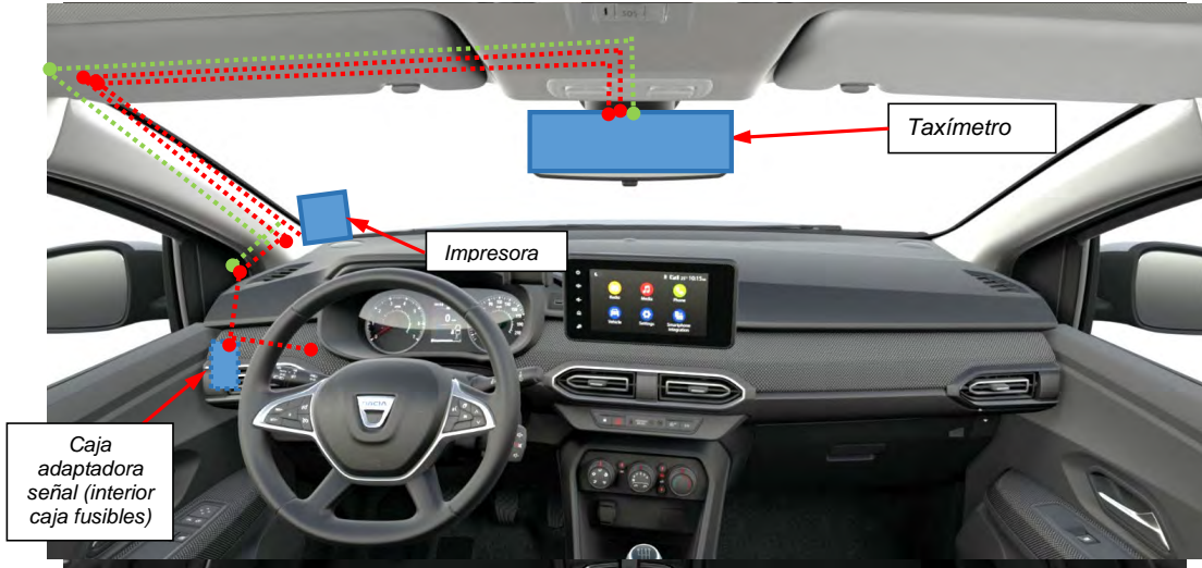
Fig. 4.4. Esquema orientativo del recorrido de las conexiones para taxímetros de espejo
