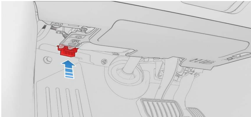
Fig. 5. Localización del conector X181
