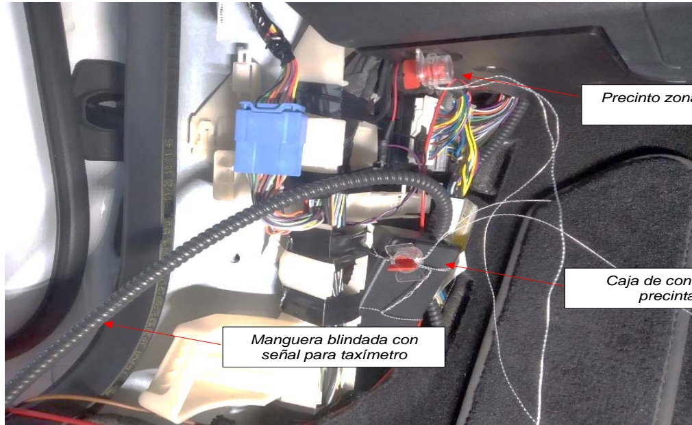
Vista final del precinto del montaje
