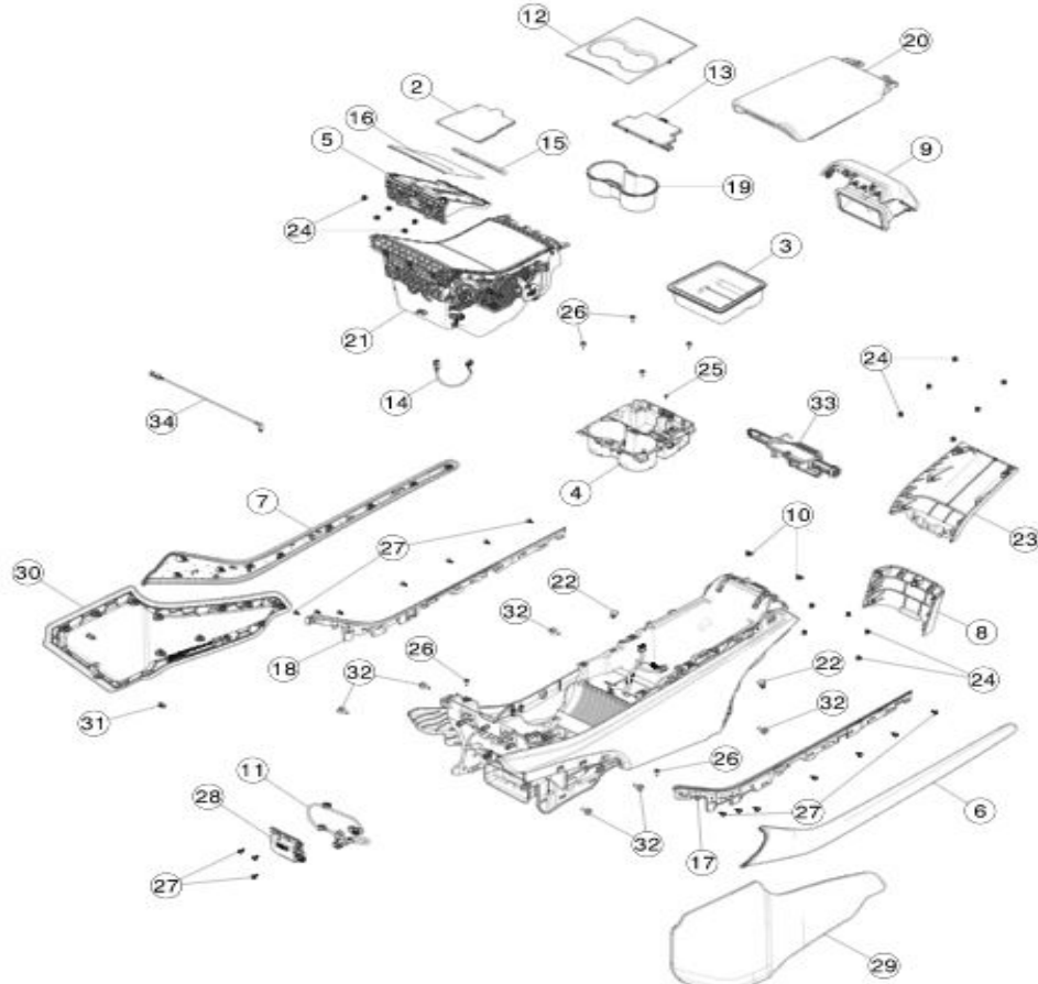
Despiece de elements de la consola central
