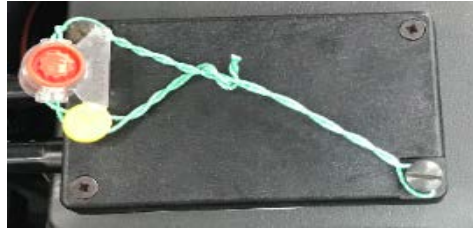
Fig. 7. Vista ejemplo de una caja de conexiones precintada
