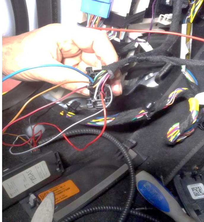
Vista de las conexiones de cables de señal y alimentación sobre el conector X181
