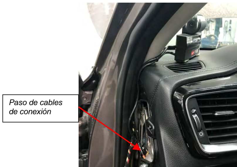
Fig. 5.3. Vistas de la conexión de la impresora.
