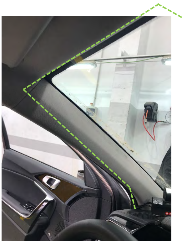
Fig. 4.3. Recorrido de los cables por el interior del guarnecido del techo
