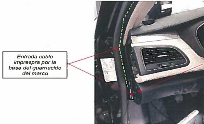
Fig. 5.8. Paso de cables de impresora del taxímetro de espejo
