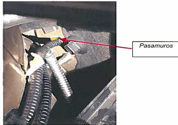
Fig. 2.3. Detalle del paso del cable de señal por el pasamuros, detrás de la zona de la guantera, vista motor
