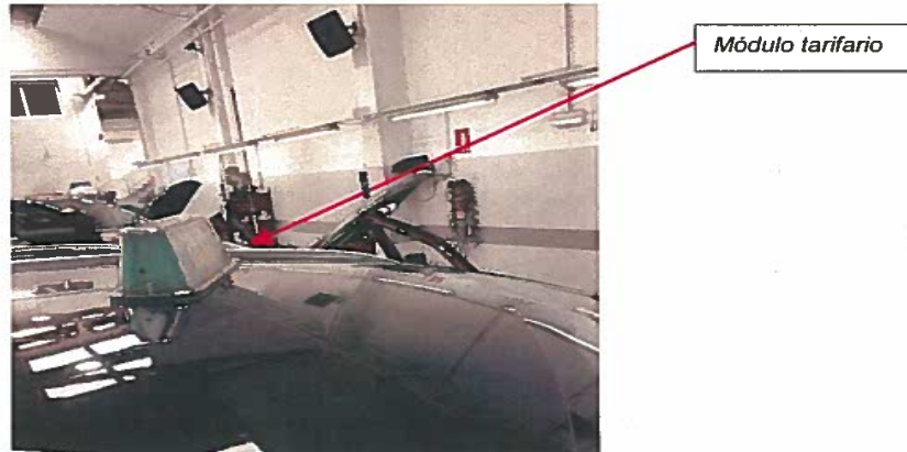
Fig. 6.1 Vista lateral del módulo atornillado
