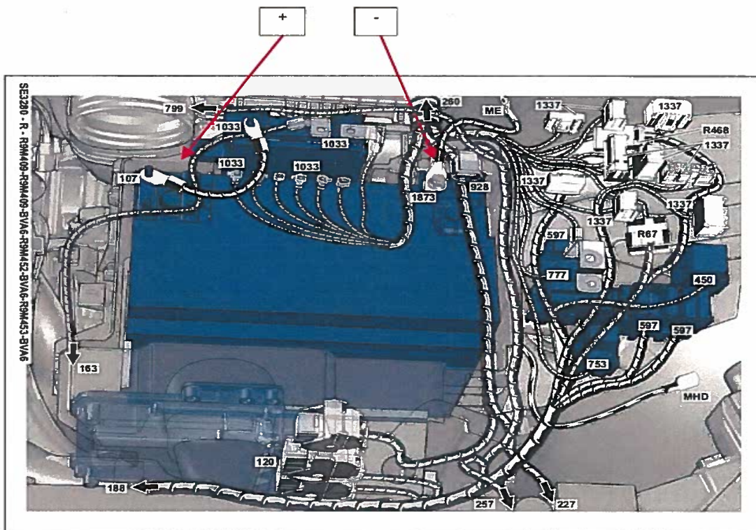
Fig. 3.1. Esquema de la batería.
