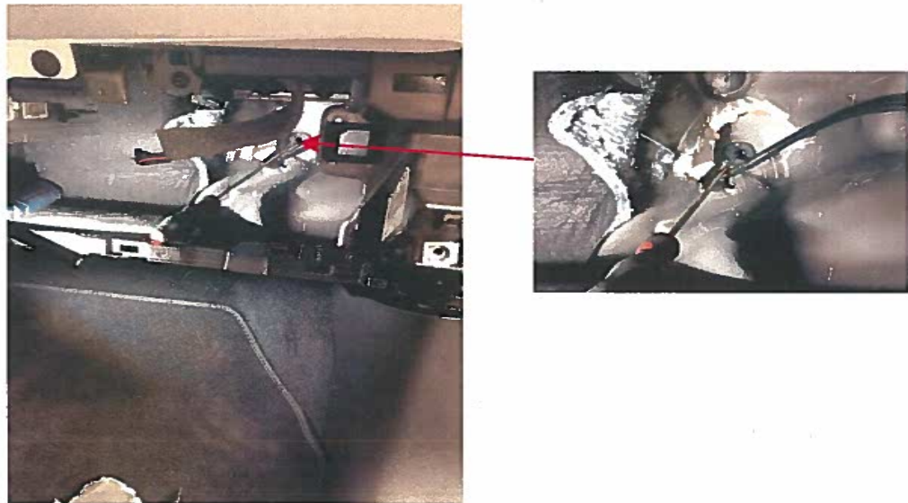
Fig. 2.4. Detalle del paso del cable de señal por el pasamuros, detrás de la zona de la guantera, vista habitáculo
