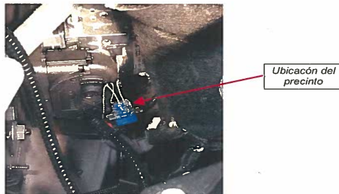
Fig. 2.2. Detalle del precintado del conector 1094 módulo ABS/ESP
