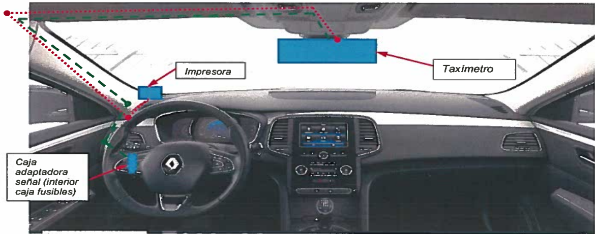
Fig. 4.4. Esquema orientativo de las conexiones para taxímetros de espejo.
