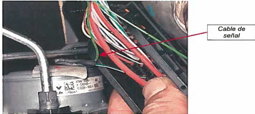
Fig. 2.1. Detalle conexión cable señal al cable del pin nº 3 del conector 1094
