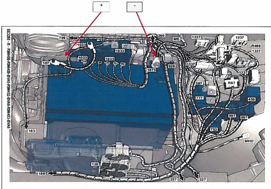
Fig. 2.1. Esquema de la batería.
