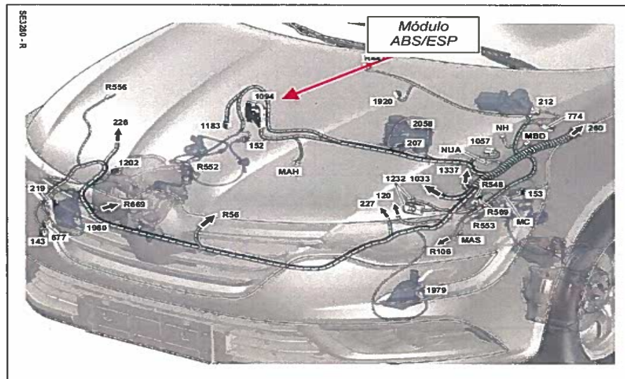
Fig. 1.2. Esquema general de conectores
