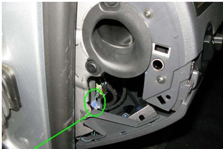
Precinto cuadro de instrumentos
