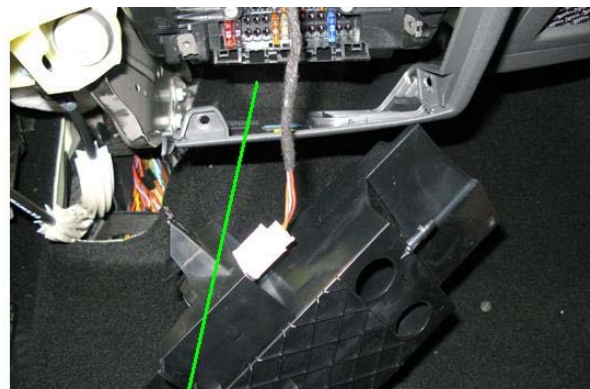
Alimentación 30 en la caja de fusibles
