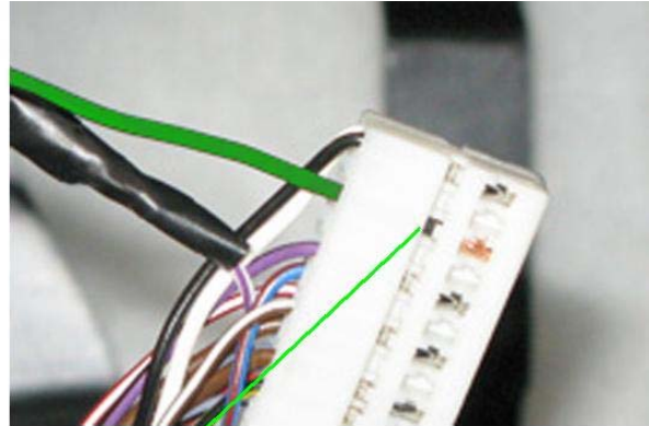
Conexión cable verde con el pin 3
