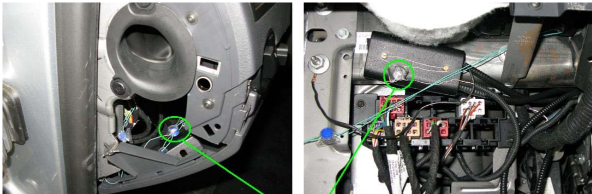
Precinto caja adaptadora
