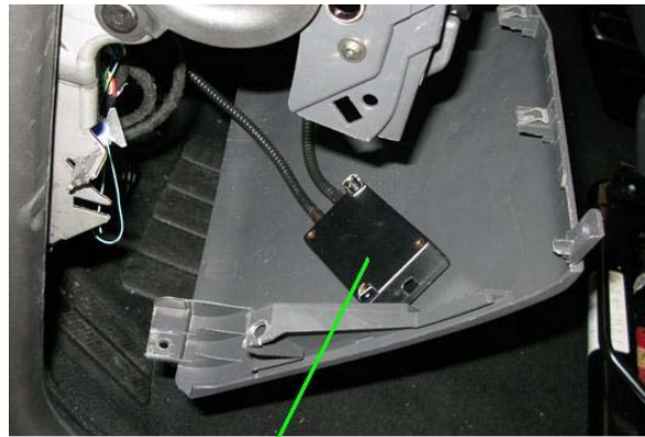
Caja adaptadora-conversora
