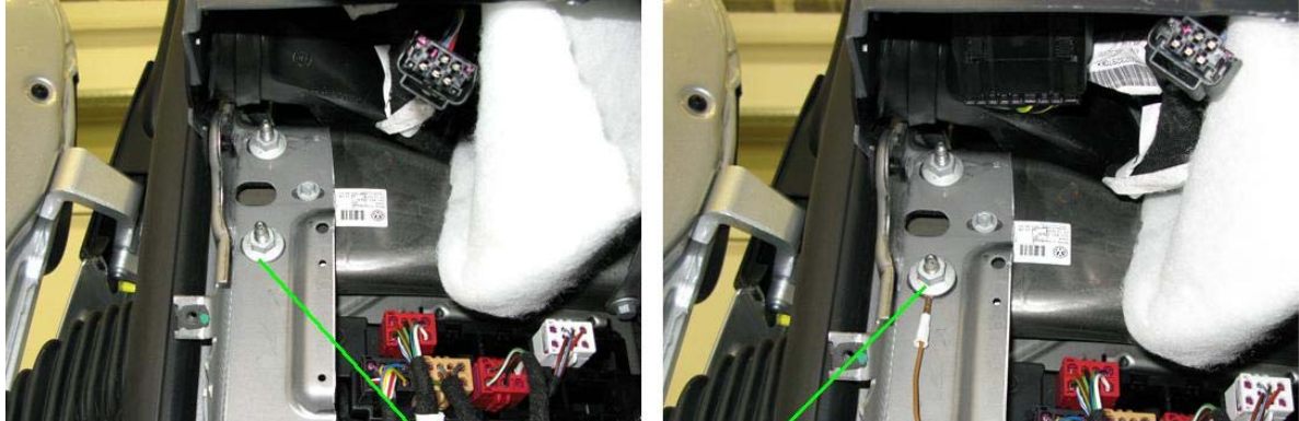
Punto de conexión (parte inferior montante A, lado conductor) de la masa
