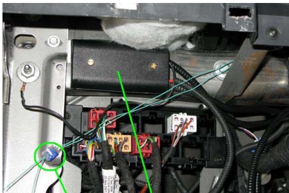
Precinto montado Caja de conexiones
